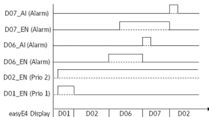
Obr. 226: Funkční diagram zobrazení textu
