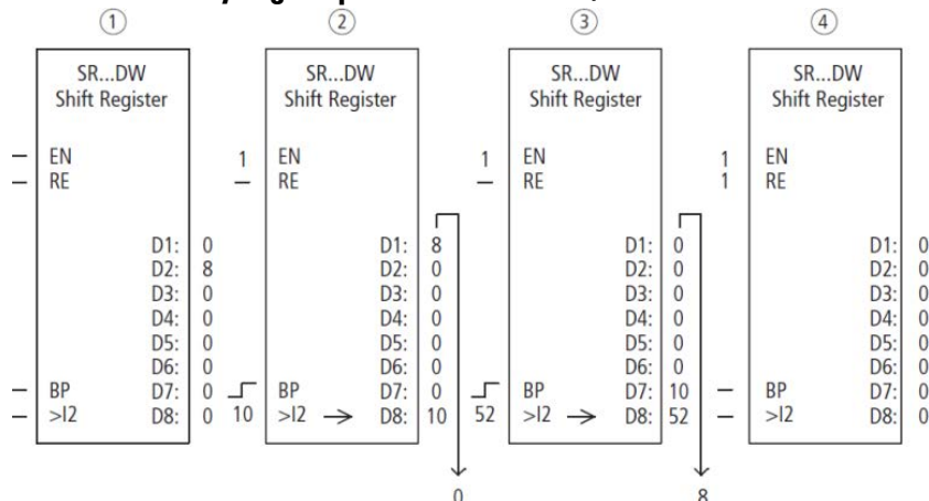
Obr. 220: Posuvný registr SR...: Zpětná operace v pracovním režimu DW
