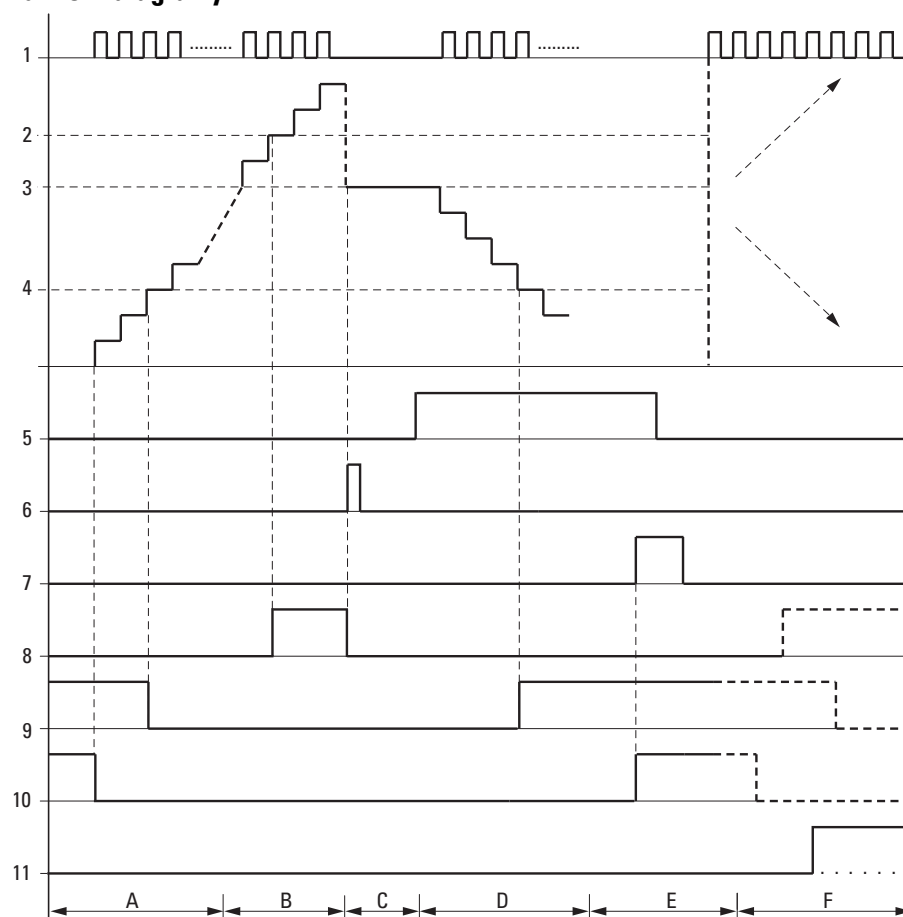
Obr. 172: Funkční diagram čítače
