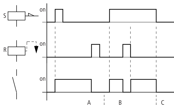
Obr. 99: Funkční diagram "Nastavit" a "Resetovat"
