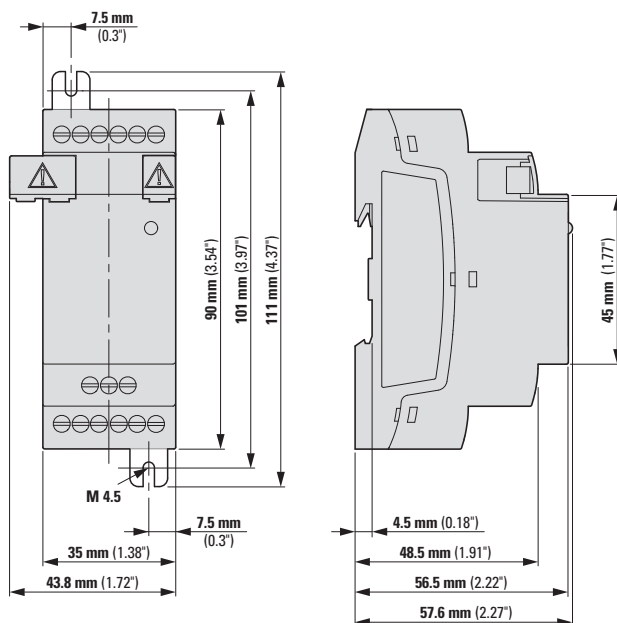
Obr. 401: Rozměry v mm (palce)
