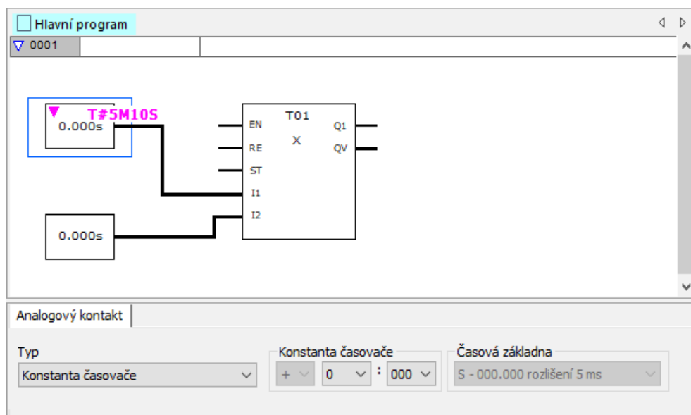
Obr. 123: Náhled programování: Vybraná konstanta časovače na vstupu modulu I1 a nepotvrzené zadání hodnoty z klávesnice <t#5m10s>
