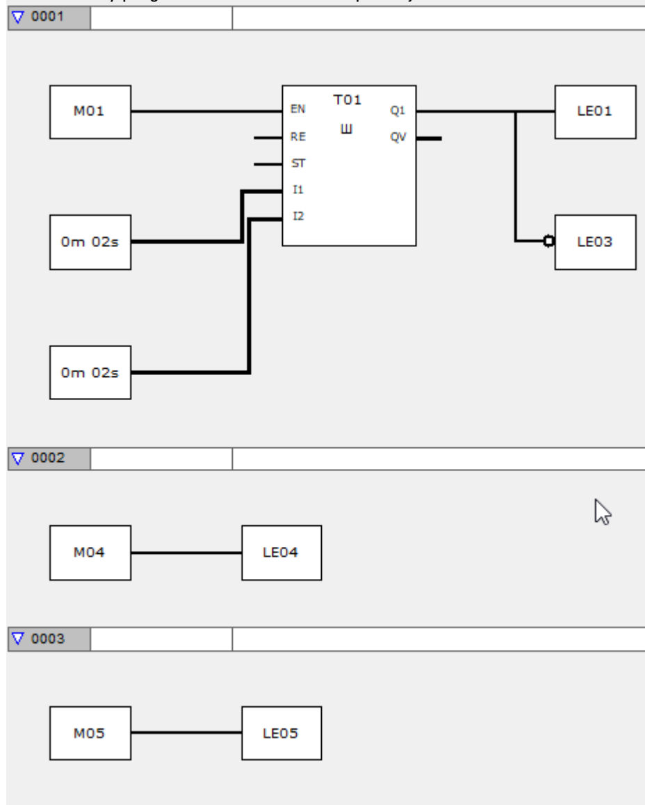
Obr. 304: Náhled programování/Příklad programu v FBD
