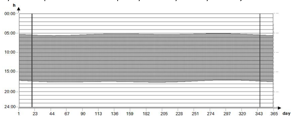
Obr. 165: Offset; O1=-2; O2=2; Q1=1 vypíná 2 hodiny před východem slunce a 2 hodiny po západu slunce
