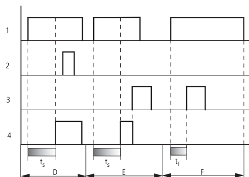
Obr. 146: Funkční diagram časového relé se zpožděnou odezvou (s náhodným spínáním a bez něj)
