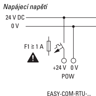
Obr. 351: EASY-COM-RTU-... Připojení napájecího zdroje
