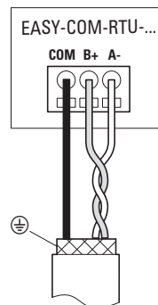
Obr. 350: EASY-COM-RTU-... Připojte výstupy
