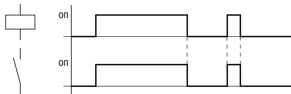
Obr. 97: Funkční diagram "Ochranná funkce"
