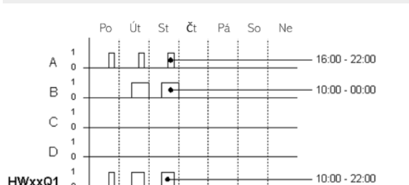
Obr. 132: Funkční diagram
