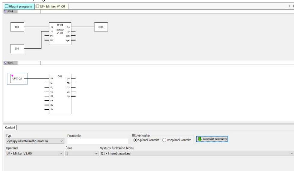
Obr. 279: Propojení vstupů/výstupů
