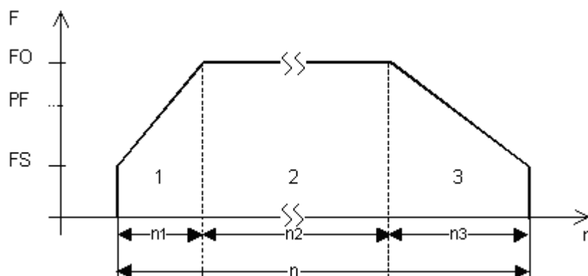
Obr. 198: Typický profil impulsu krokového motoru v normálním provozu
