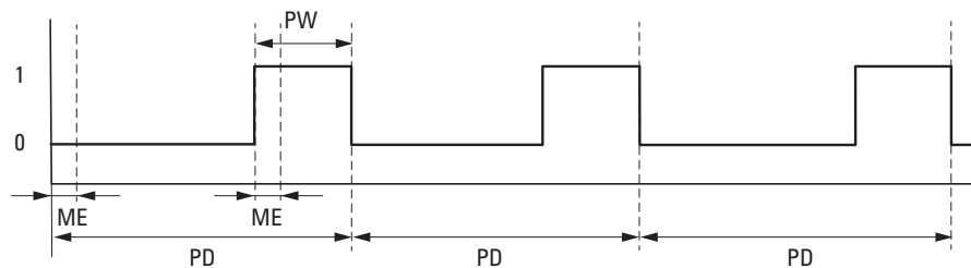
Obr. 189: Impulsy PW na vstupu modulu při SV = 1400 , ME = 93 ms, PD = 1000 ms
