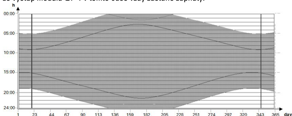
Obr. 170: Q1 nevypne v průběhu letních měsíců
