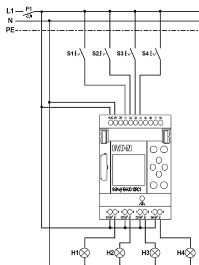
Obr. 405: Spínací schéma indikátoru easy4
