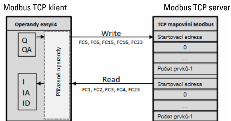
Obr. 389: Přehled funkčního kódu cyklických dat
