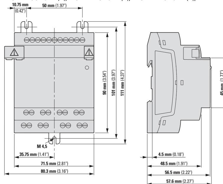
Obr. 399: Rozměry v mm (palce) rozšíření 4TE
