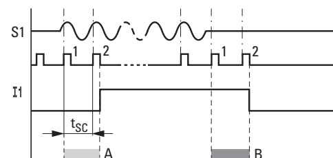
Obr. 310: Chování při sepnutí vstupního signálu AC při aktivním snížení odskoku I
