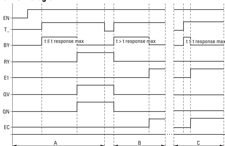
Obr. 242: Funkční diagram frekvenčního čítače
