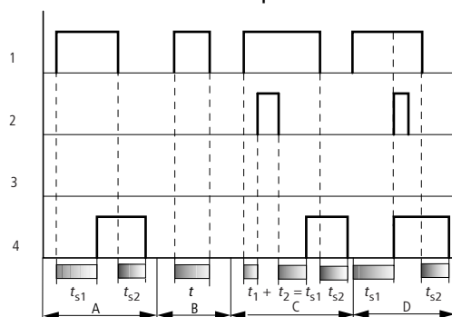
Obr. 149: Funkční diagram časového relé, se zpožděnou odezvou a zpožděným odpadem
