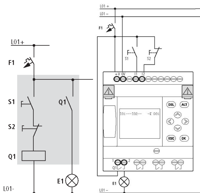
Obr. 83: Ovládání žárovek
