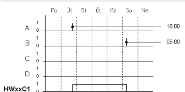
Obr. 130: Funkční diagram
