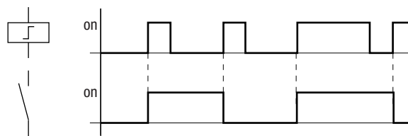
Obr. 98: Funkční diagram "Impulzní relé"
