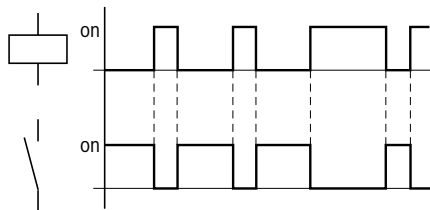
Obr. 101: Funkční diagram "Inverzní funkce stykače"
