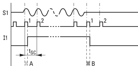
Obr. 311: Chování vstupního signálu AC při neaktivním snížení odskoku I
