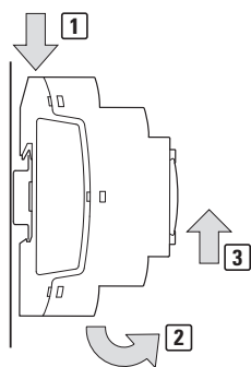
Obr. 16: Demontáž
