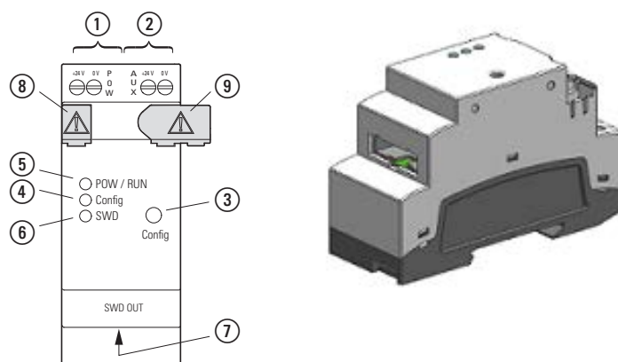
Obr. 344: Provedení přístroje v 2TE
