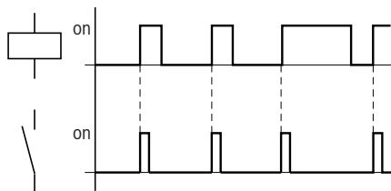
Obr. 102: Funkční diagram "Impulz cyklu" při kladném náběhu
