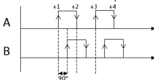
Obr. 175: Funkční blok CI počítán vzestupně; QV=QV+4
