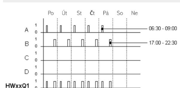
Obr. 128: Funkční diagram
