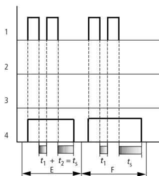
Obr. 148: Funkční diagram časového relé, se zpožděným odpadem (s/bez náhodného sepnutí, s/bez opětovného spouštění)
