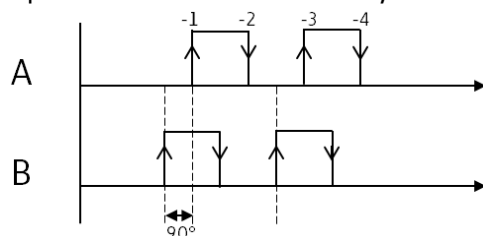
Obr. 176: Funkční blok CI počítán sestupně; QV=QV-4
