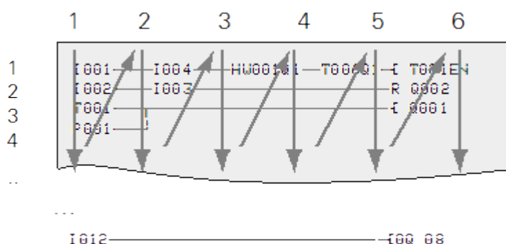
Obr. 303: Jak easyEDP vyhodnocuje spínací schéma
