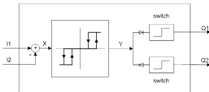
Obr. 203: Princip zapojení tříbodového regulátoru
