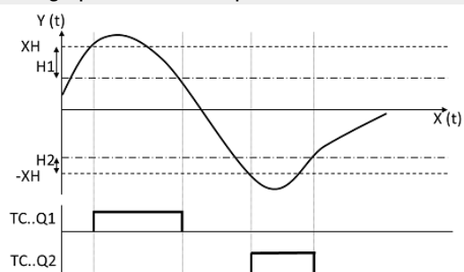
Obr. 205: Funkční diagram tříbodového regulátoru
