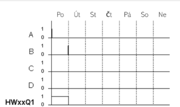
Obr. 134: Funkční diagram
