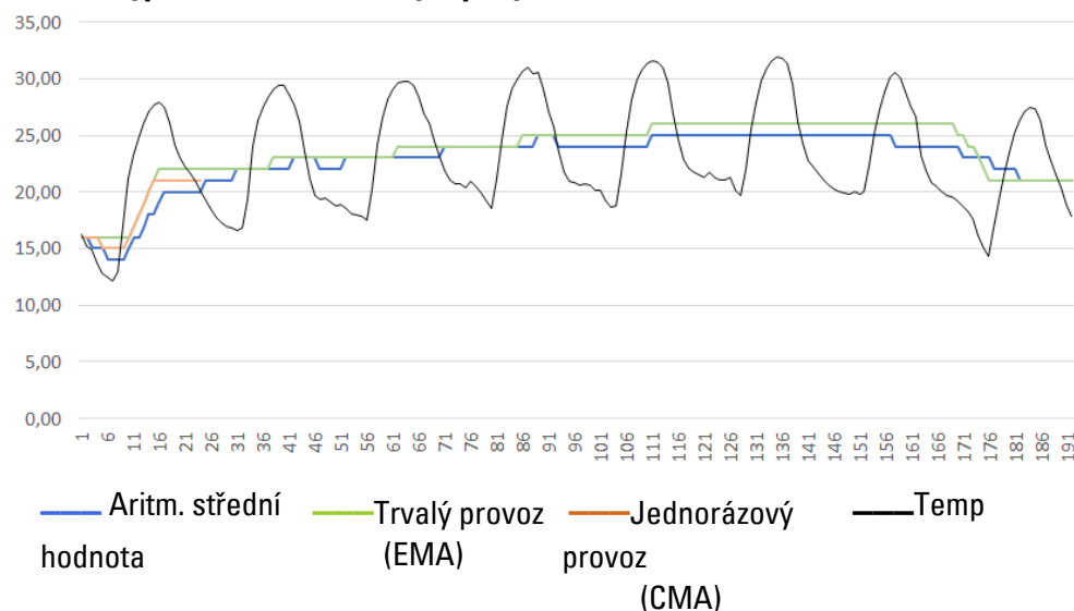
Obr. 182: Příklad charakteristiky snímání teploty jednou za hodinu, po 7 dnů
