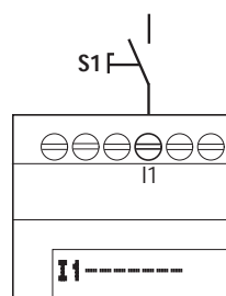
Obr. 306: Obsazení vstupu easyE4 spínačem
