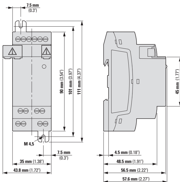
Obr. 400: Rozměry v mm (palce) rozšíření 2TE
