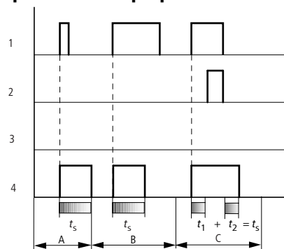
Obr. 150: Funkční diagram časového relé, podle impulsu 1
