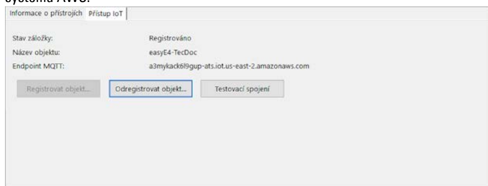
Obr. 367: Odhlášení easyE4
