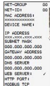
Informace\Actual Config
