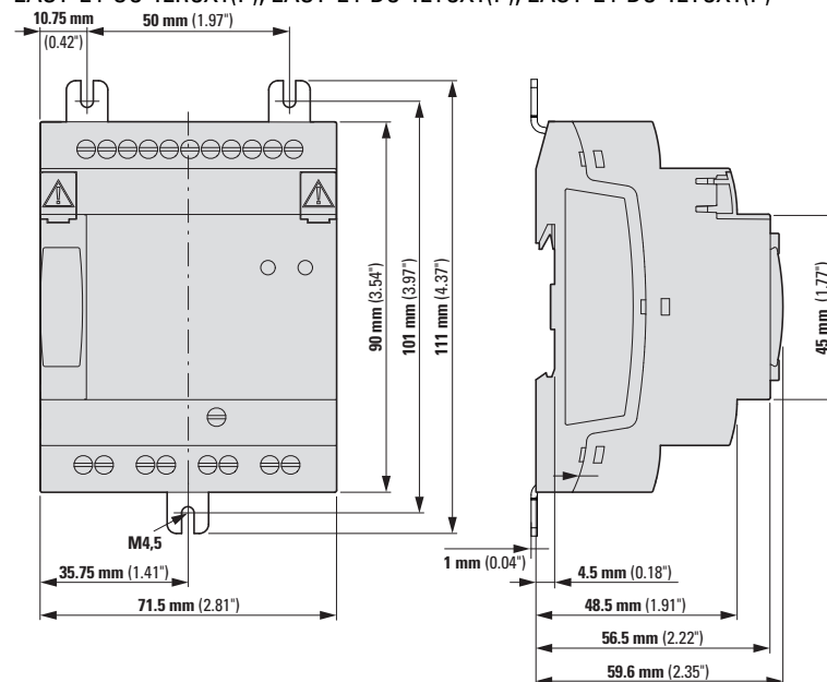
Obr. 398: Rozměry v mm (palce) základních přístrojů EASY-E4-...-12...CX1(P)
