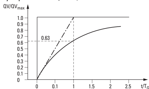
Obr. 195: Skoková odezva modulu FT
