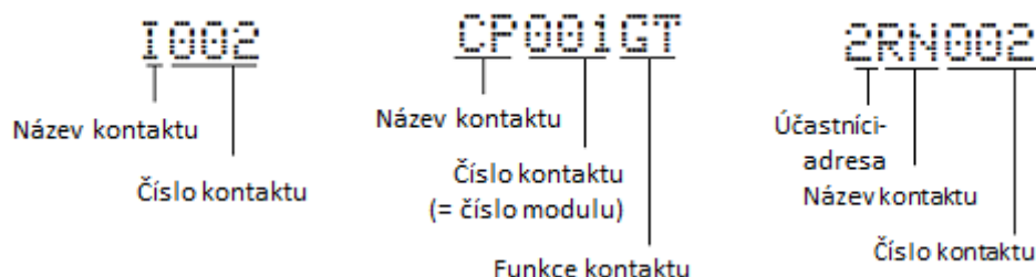
Obr. 105: Legenda zobrazení kontaktů
