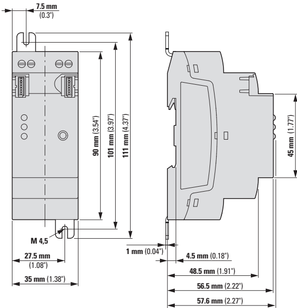
Obr. 402: Rozměry v mm (palce) rozšíření 2TE
