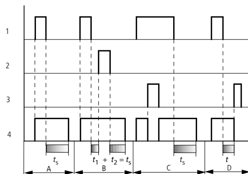
Obr. 147: Funkční diagram časového relé, se zpožděným odpadem (s/bez náhodného sepnutí, s/bez opětovného spouštění)
