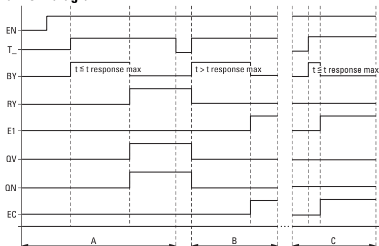
Obr. 252: Funkční diagram frekvenčního čítače
