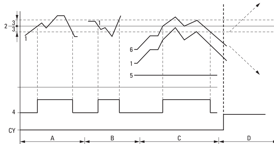
Obr. 178: Pracovní diagram analogového komparátoru
