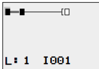
Obr. 90: Zobrazení se zvětšením, tok proudu přerušeny
