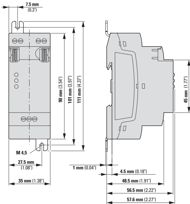
Obr. 403: Rozměry v mm (palce) rozšíření 2TE
