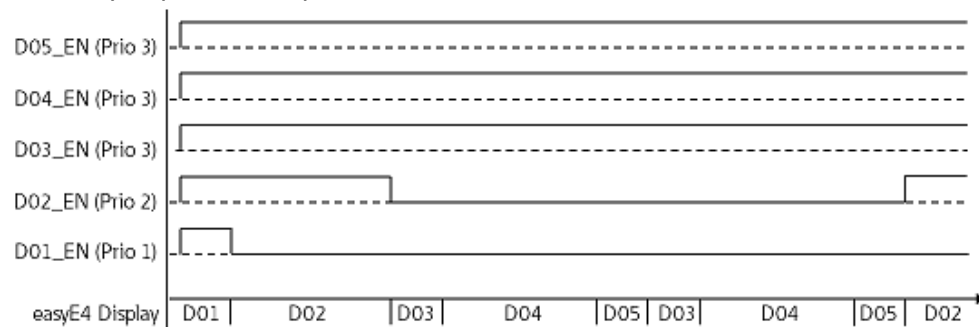
Obr. 227: Funkční diagram zobrazení textu s textovými moduly se stejnou prioritou 3
