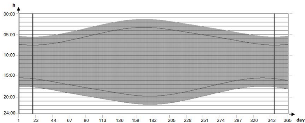
Obr. 168: Offset; O1=-2; O2=2; Q1=1 vypíná 2 hodiny před východem slunce a 2 hodiny po západu slunce
