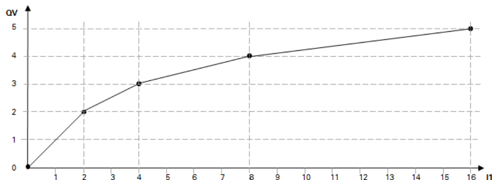
Obr. 188: Příklad charakteristiky pro funkční blok PM
