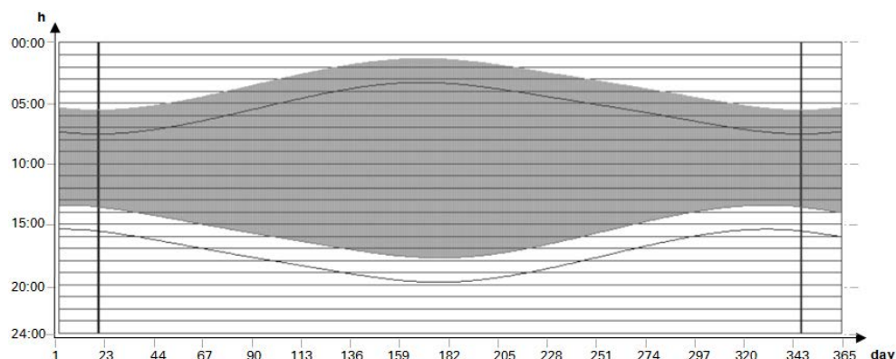
Obr. 169: Offset; O1=-2; O2=-2; Q1=1 vypíná 2 hodiny před východem slunce a 2 hodiny před západem slunce
