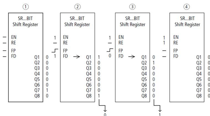
Obr. 219: Posuvný registr SR...: Dopředná operace v pracovním režimu BIT
