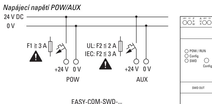
Obr. 345: EASY-COM-SWD-... Připojení napájecího zdroje
