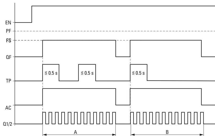
Obr. 200: Funkční diagram krokovací provoz s předem zadaným počtem kroků P1
