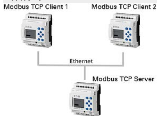
Obr. 383: Příklad: easyE4 jako server Modbus TCP
