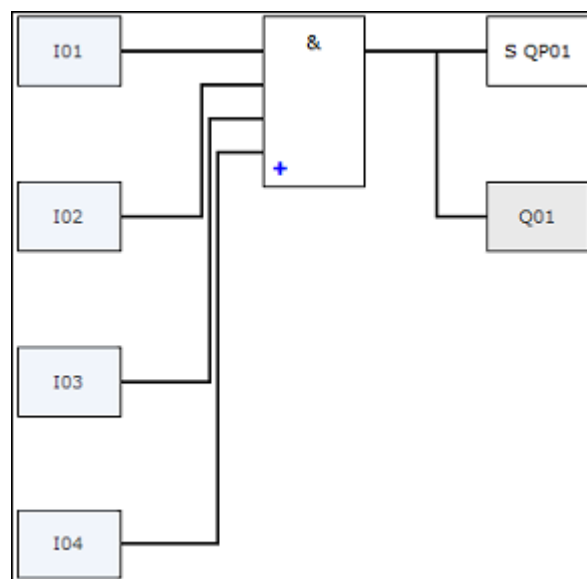
Obr. 269: Předání stavů ze vstupů a výstupů mezi hlavním programem a programem přerušení
