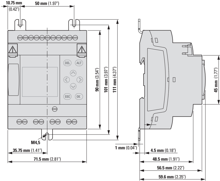
Obr. 397: Rozměry v mm (palce) základních přístrojů EASY-E4-...-12...C1(P)
