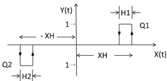
Obr. 204: Časový diagram tříbodového regulátoru
