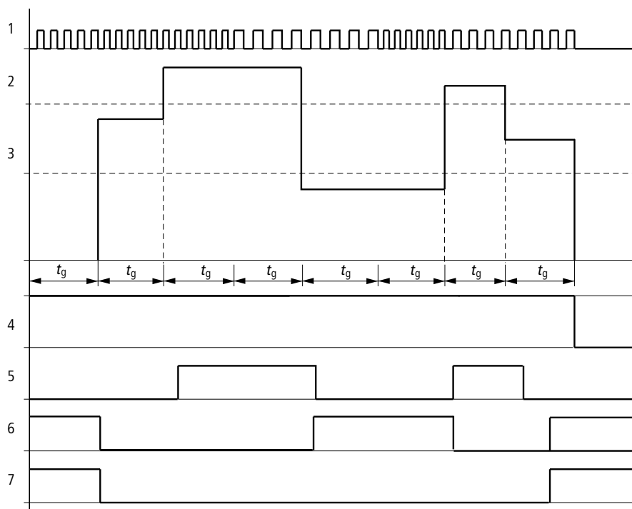
Obr. 173: Funkční diagram frekvenčního čítače
