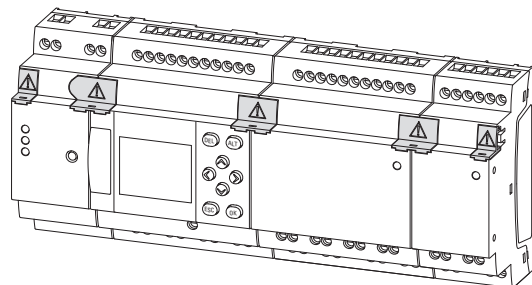
Obr. 343: Příklad řídicího relé easyE4 s rozšířeními I/O a komunikačním modulem easy EASY-COM-SWD-...
