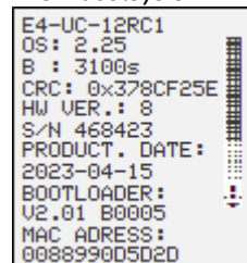
Informace\Systém
