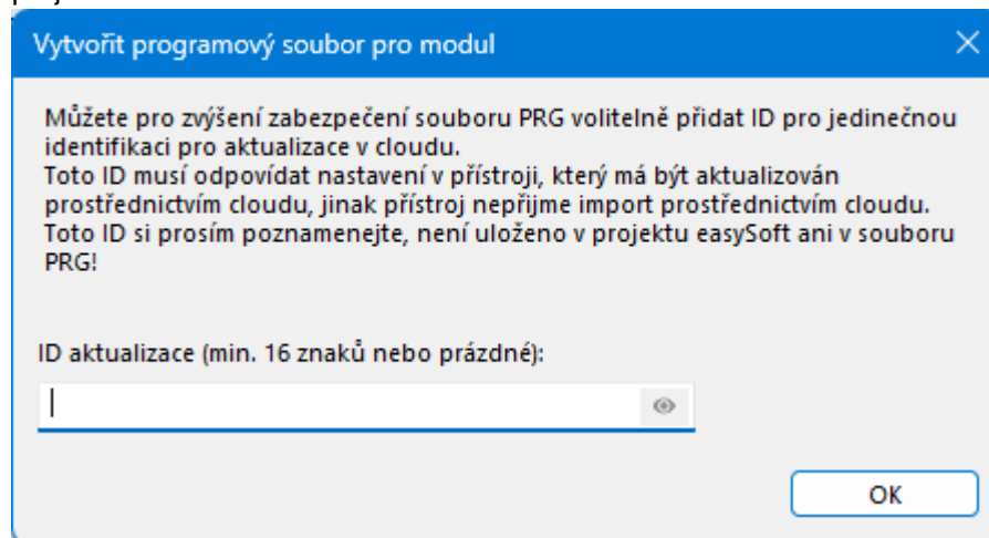
Obr. 380: ID aktualizace
