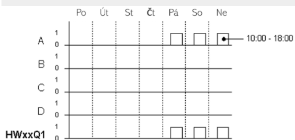
Obr. 126: Funkční diagram
