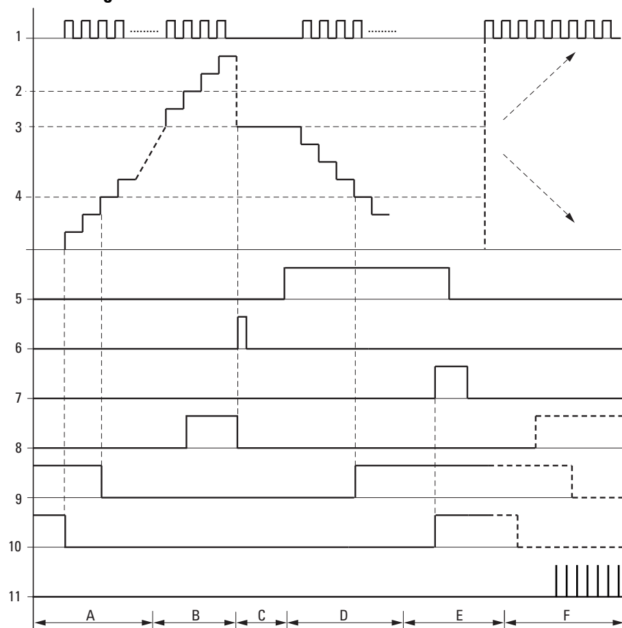
Obr. 177: Funkční diagram rychlého inkrementálního čítače
