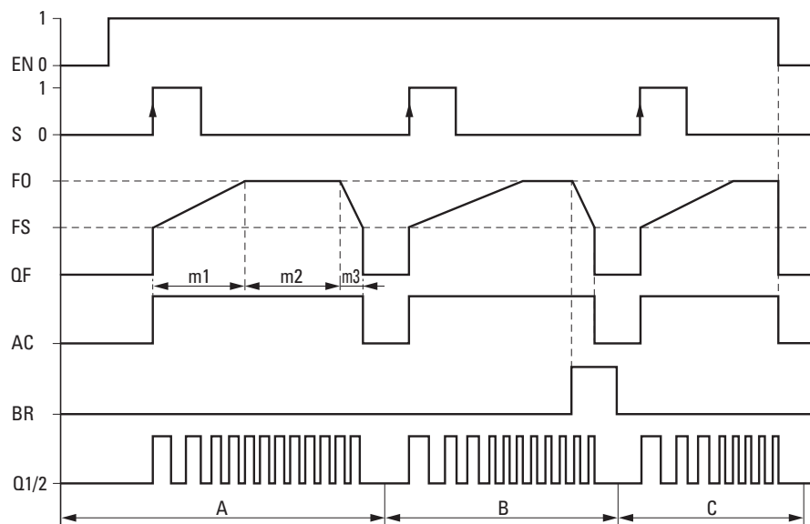
Obr. 199: Funkční diagram výstup impulsu PO při předem zadaném počtu impulsů I1 - možné fáze normálního provozu
