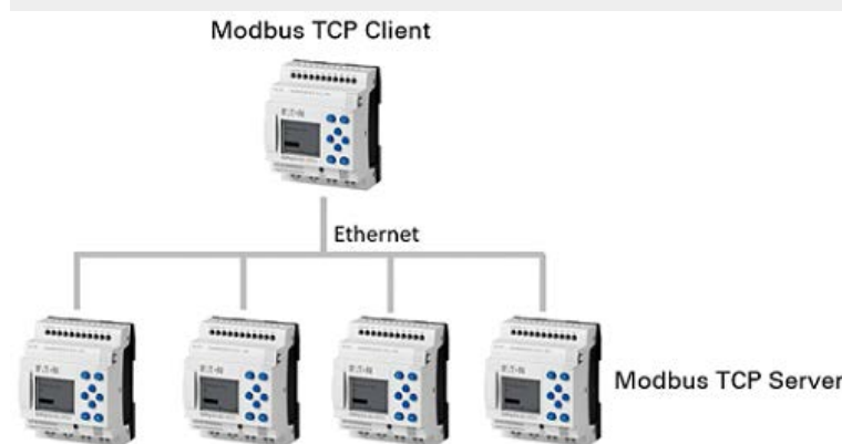
Obr. 382: Příklad: easyE4 jako klient Modbus TCP
