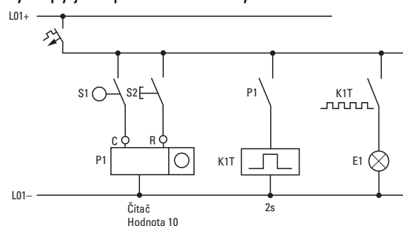
Obr. 290: Pevné zapojení s relé
