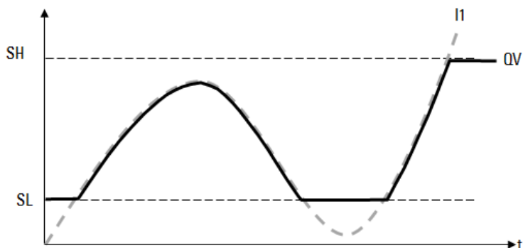
Obr. 206: Obr.: Ořezání vstupních hodnot na pevně stanovených hranicích
