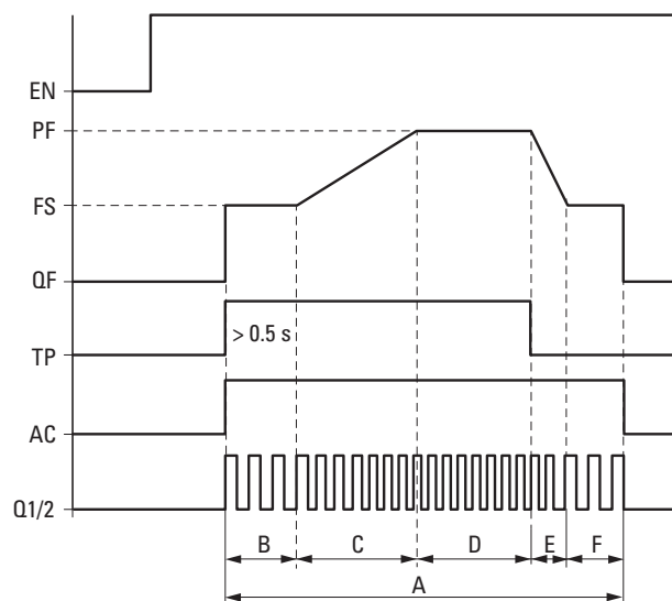
Obr. 202: Funkční diagram krokovací provoz s předem zadanou krokovací frekvencí, P1 není dosaženo po fázi brždění
