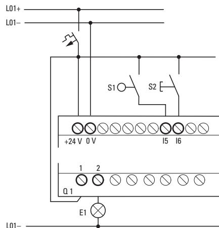
Obr. 291: Zapojení například s EASY-E4-UC-...
