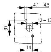
Drilling dimensions door
