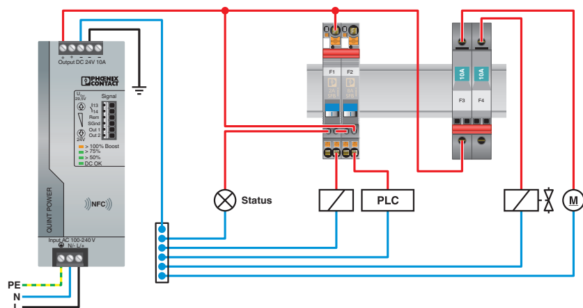
applicatietekening
