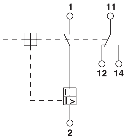
schakelschema
