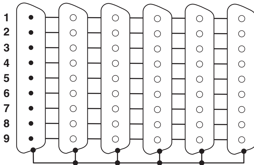
schakelschema
