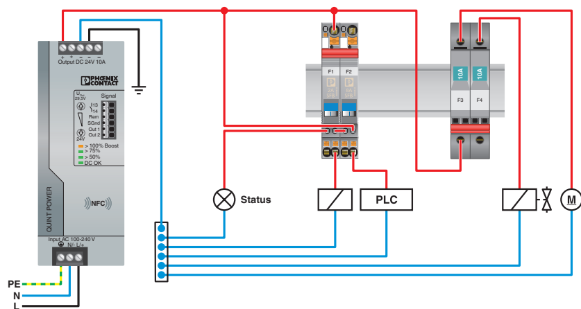
applicatietekening
