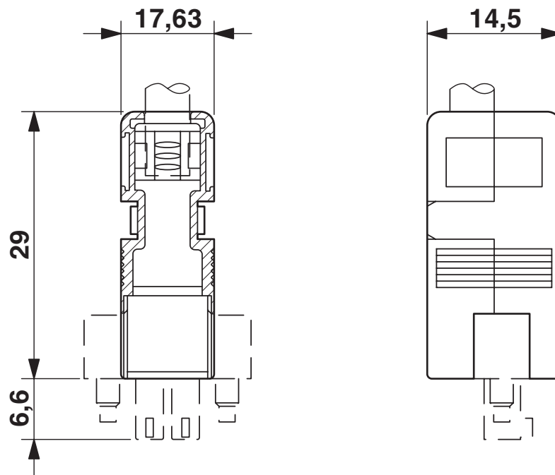
Maatschets
