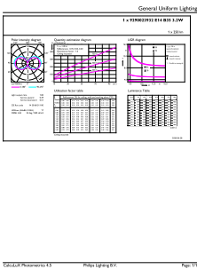
LEDbulb CLA 3,2W B35 E14 927 922 CL
