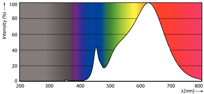
LEDbulb CLA 3,2W B35 E14 927 922 CL
