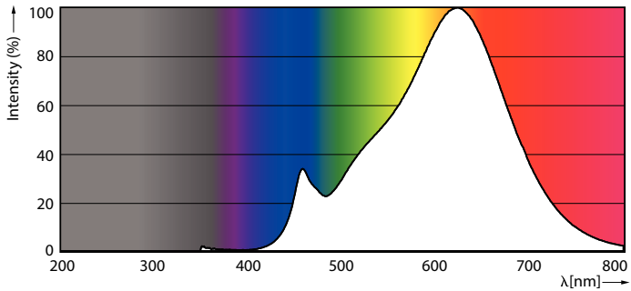
LEDbulb CLA 4,5W BA35 E14 927 922 CL
