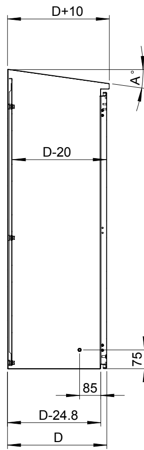
SECTION A-A
