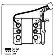
Wiring
