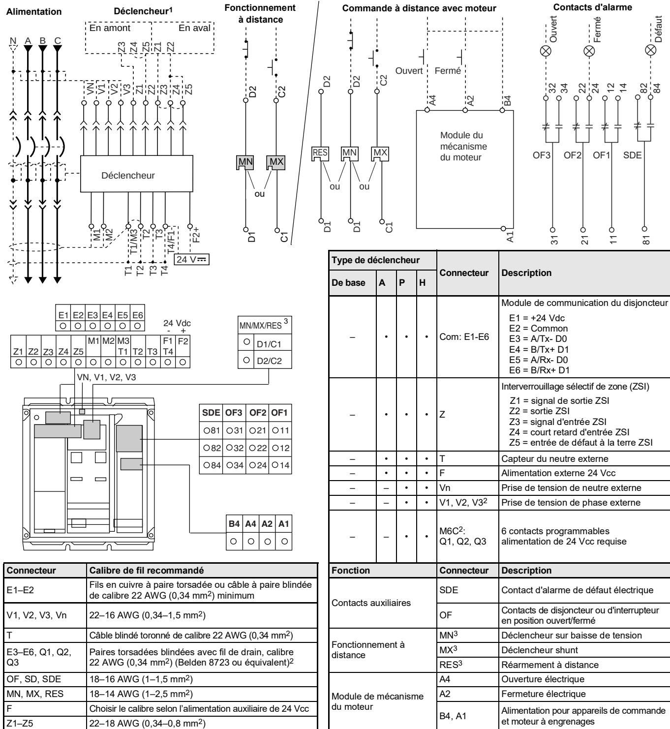
FIG. 5 : Schémas de câblage de commande des accessoires (Français)
