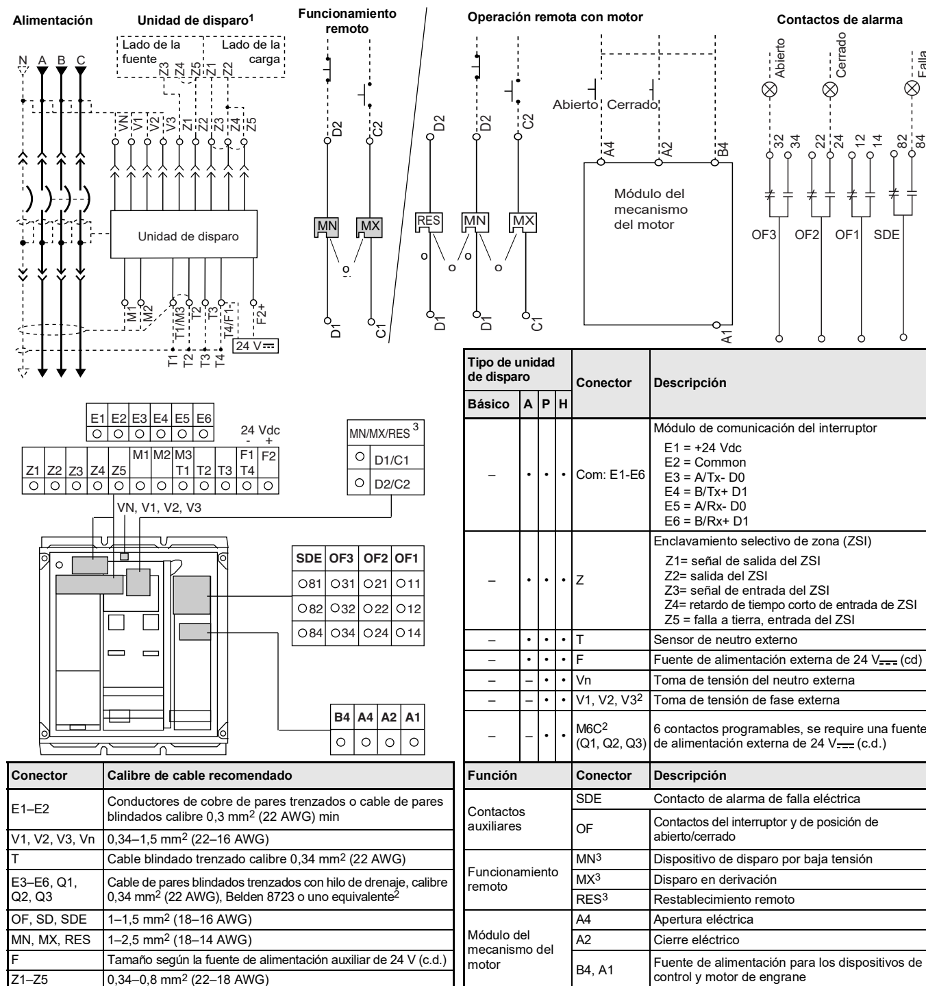
FIG. 4 : Diagramas del cableado de control de los accesorios (Español)
