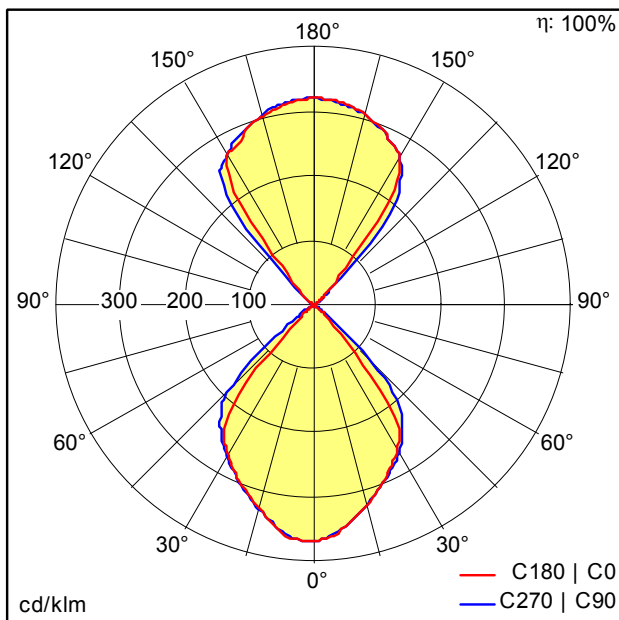
TE_HOLLY_CONE_UPDOWN_IP65_500_830.ltd
