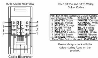
Wiring
