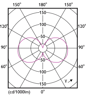
LEDcandle MAS SLR B35 3,4W E14 927 CL-LDD
