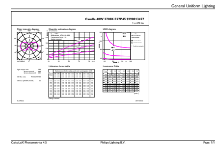
LEDbulb 40W E27 827 FR P45
