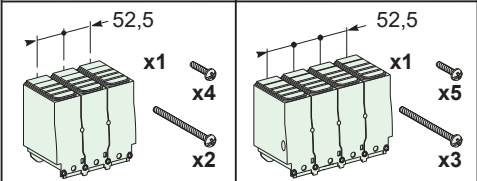
3P LV432595
