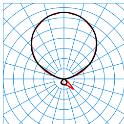
Luceos S-T PAW-IL 300-830 ETDD 03 (LEO1) TX245494
