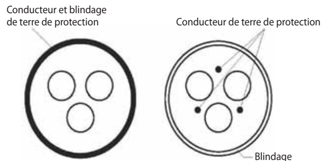
Figure 28. Description du câble
