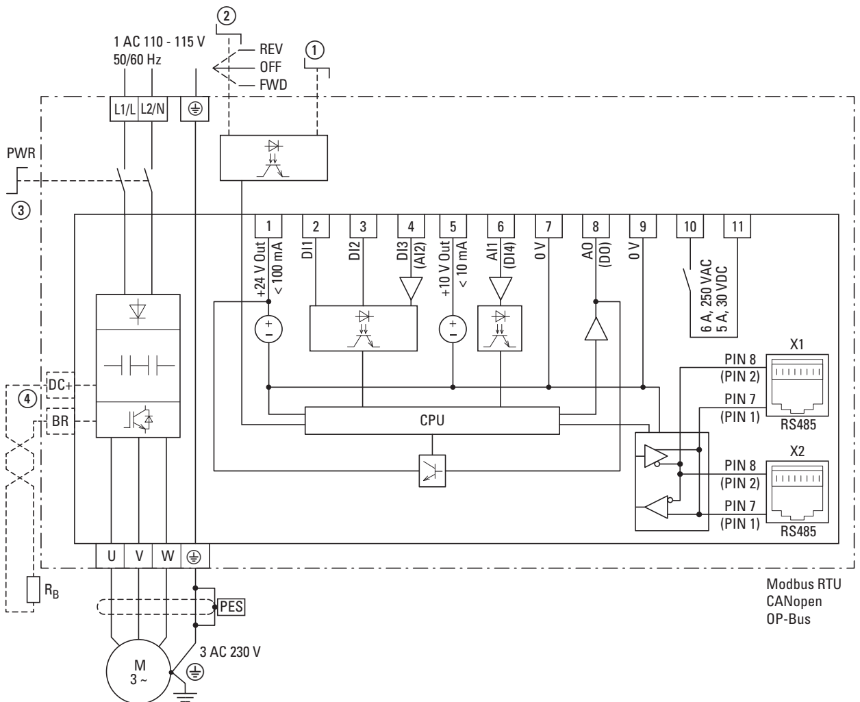
Abbildung 66: Blockschaltbild DC1-1D...Nx-A6S...
