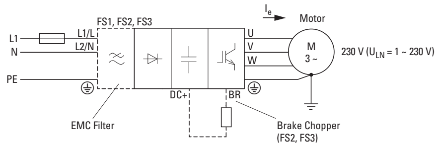
Abbildung 9: DC1-12...
