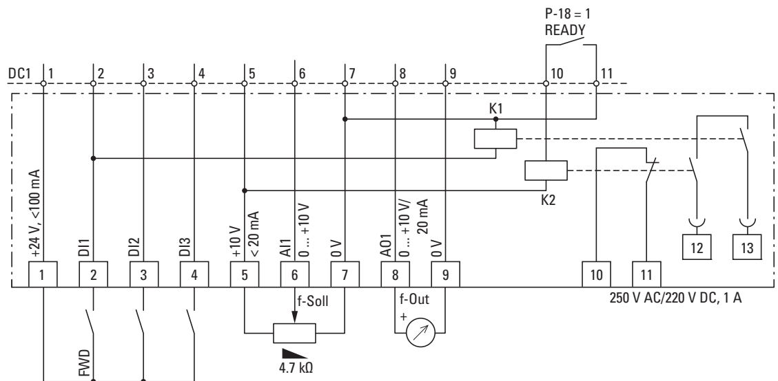
Abbildung 92: Blockschaltbild DXC-EXT-2RO1AO
