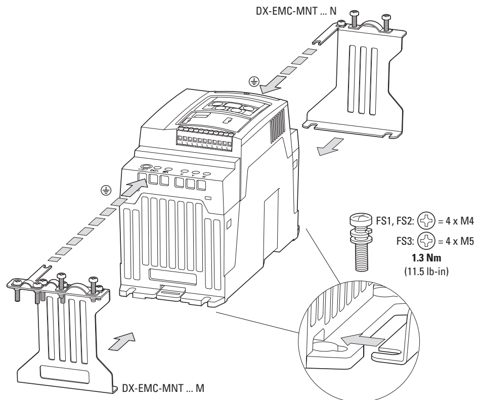
Abbildung 40: EMV-Kabelhalterungen (Beispiel: Baugröße FS2)
