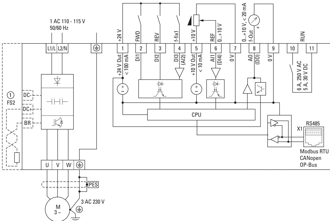
Abbildung 62: Blockschaltbild DC1-1D...Nx...
