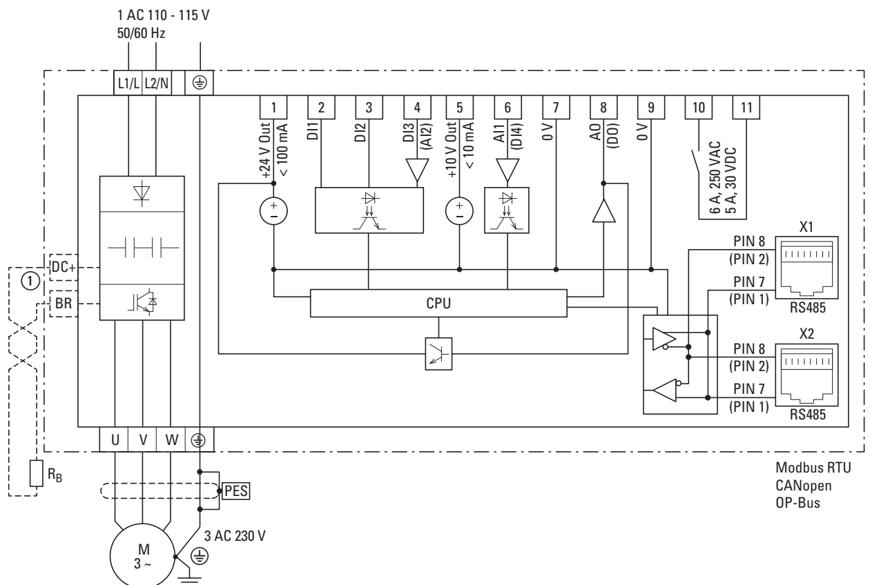
Abbildung 67: Blockschaltbild DC1-1D...Nx-A66...
