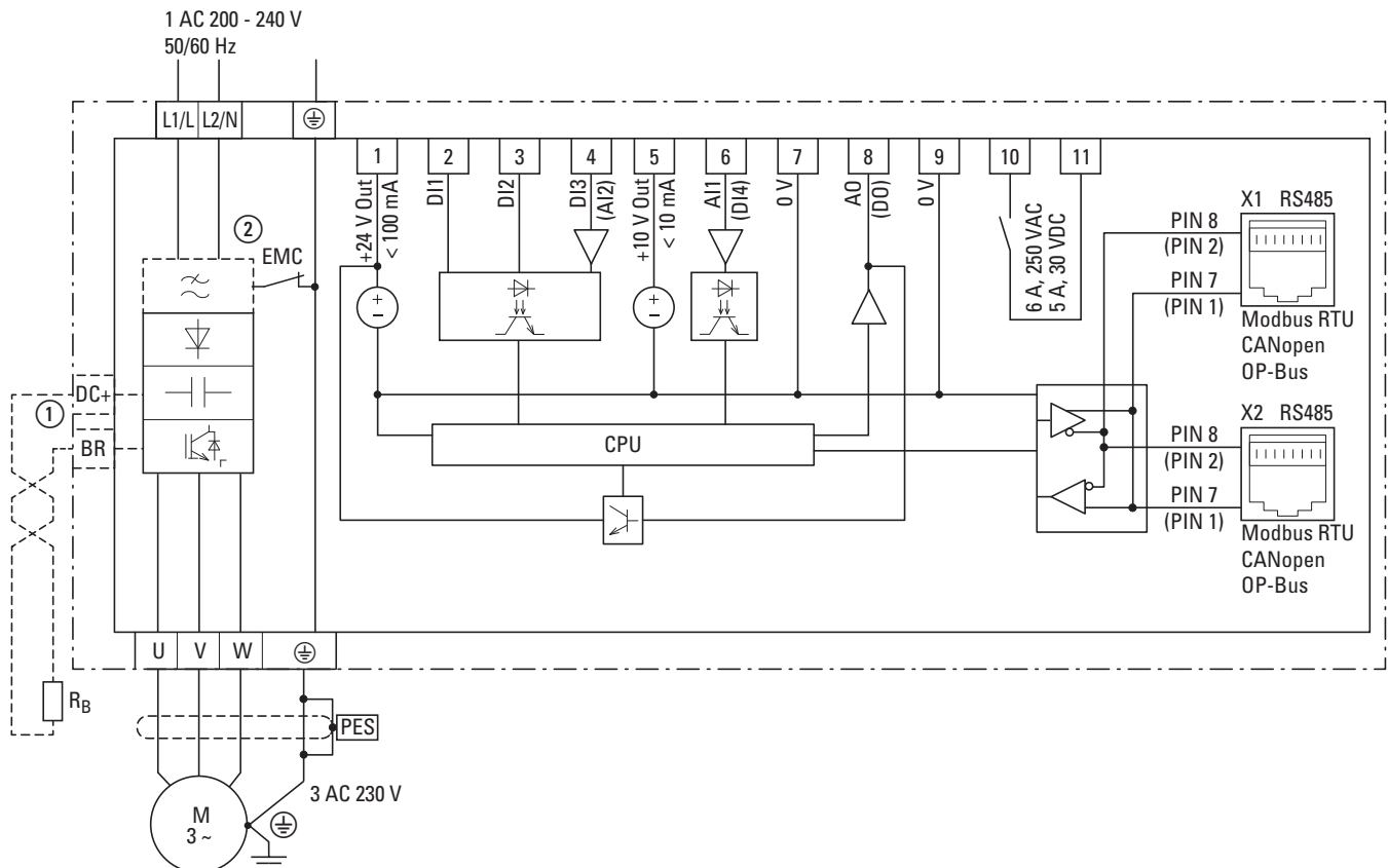
Abbildung 69: Blockschaltbild DC1-12...-A66...
