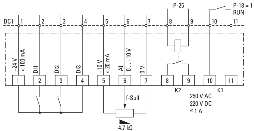
Abbildung 90: Blockschaltbild DXC-EXT-2RO
