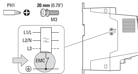
Abbildung 36: EMC-Schraube
