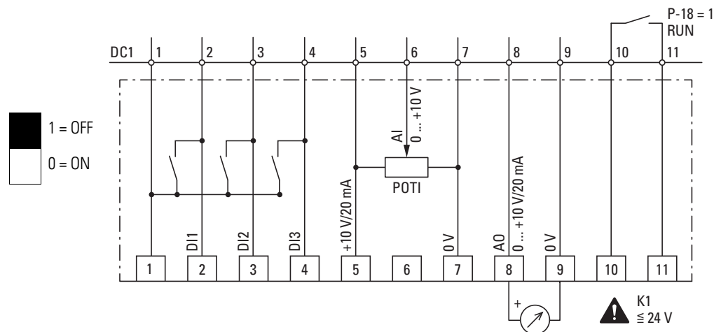
Abbildung 94: Blockschaltbild Simulator DXC-EXT-LOCSIM
