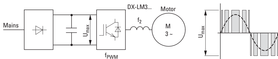
Abbildung 17: Bemessungsdaten DX-LM3...:
