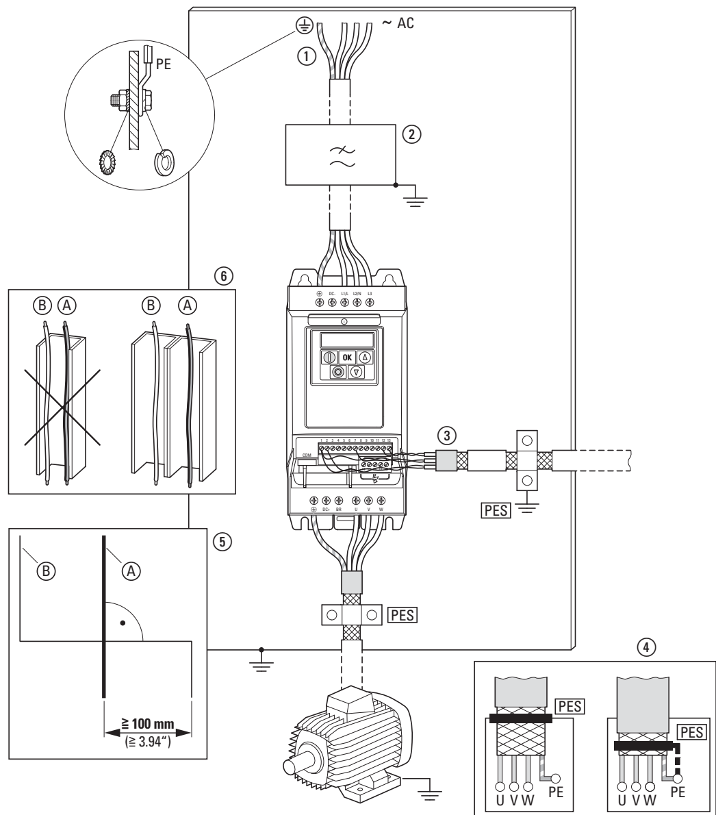
Abbildung 41: EMV-gerechte Installation
