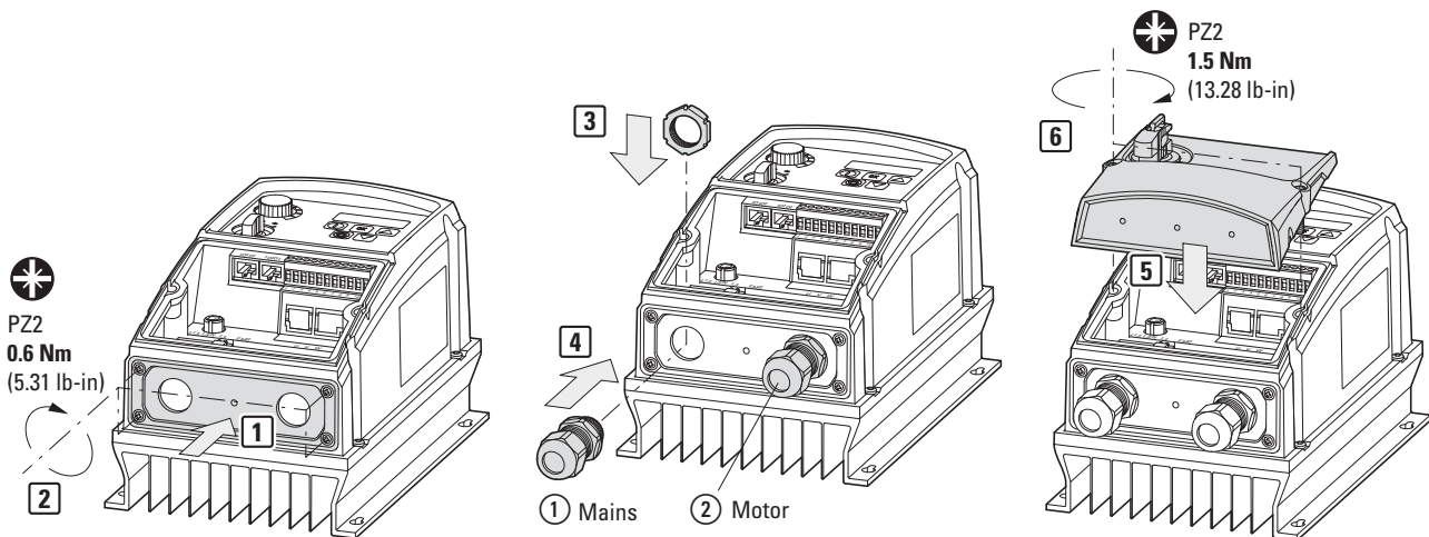
Abbildung 50: Kabelverschraubungen montieren.
