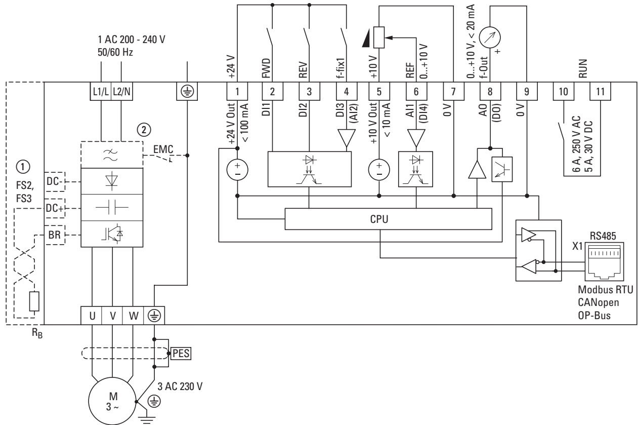
Abbildung 63: Blockschaltbild DC1-12...
