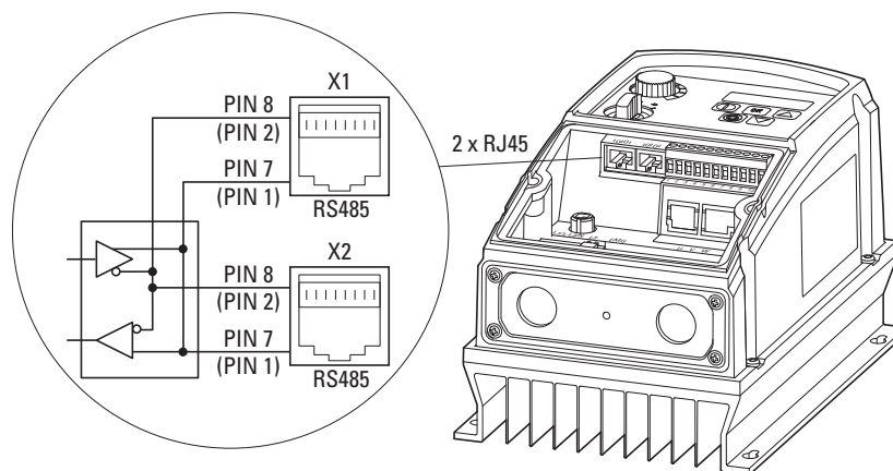
Abbildung 60: RJ45-Schnittstellen (IP66)
