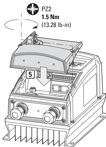
Abbildung 43: Untere Gehäuseabdeckung entfernen
