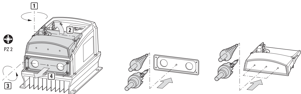
Abbildung 49: Bohrungen
