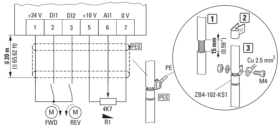
Abbildung 53: Einfaches Anschlussbeispiel
