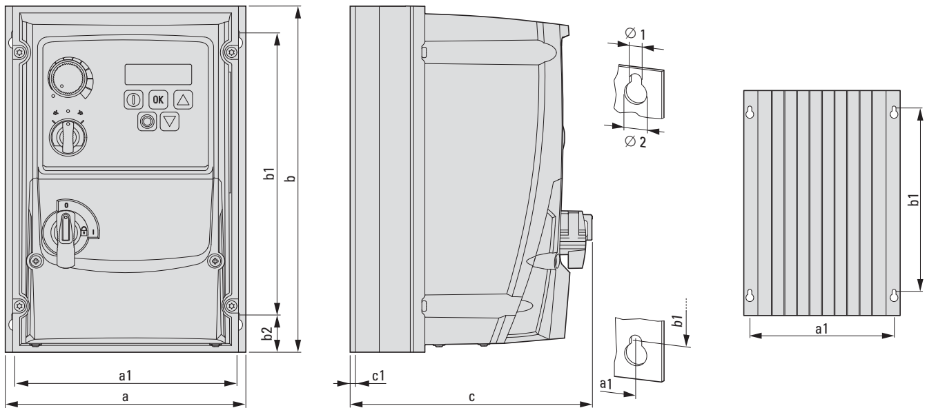
Abbildung 78: Abmessungen DC1 in Schutzart IP66 (NEMA 4X)
