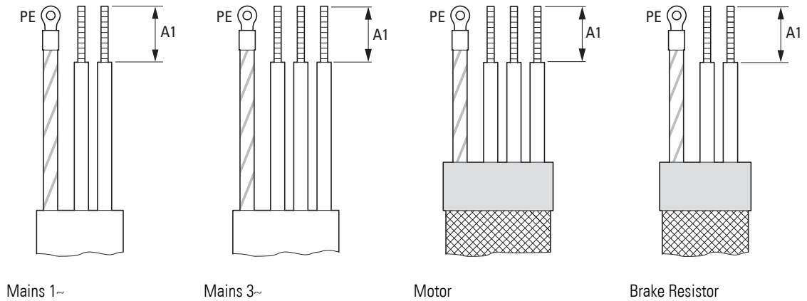
Abbildung 45: Abisolierlängen im Leistungsteil
