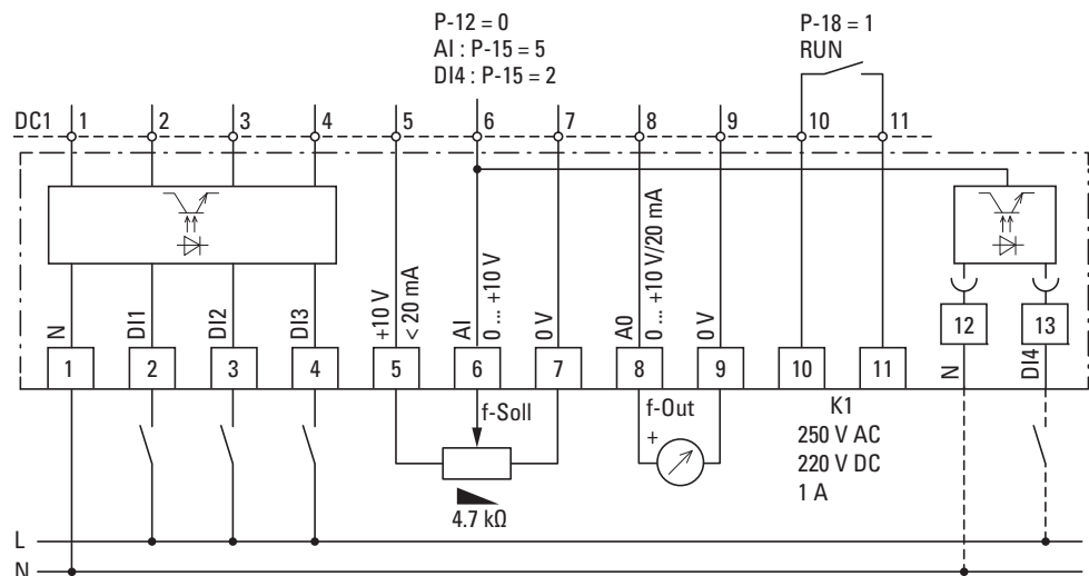
Abbildung 88: Blockschaltbild DXC-EXT-IO110 und DXC-EXT-IO230
