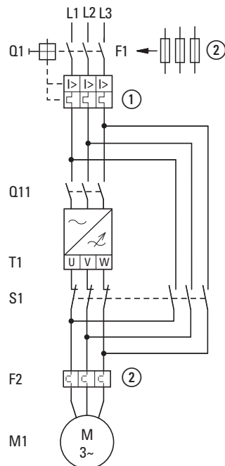
Abbildung 18: Bypass-Motorsteuerung (Beispiel)
