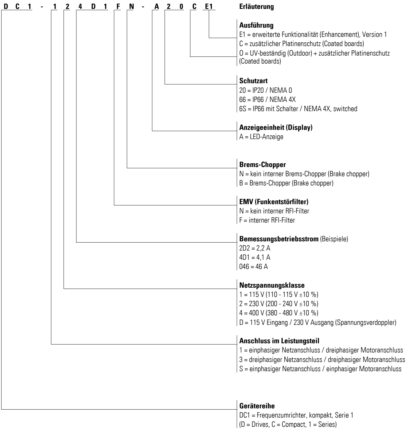
Abbildung 5: Typenschlüssel
