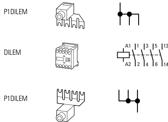
Abbildung 79: Netzschütz bei einphasigem Anschluss (DC1-12...)
