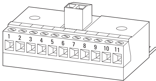
Abbildung 87: DXC-EXT-IO110 und DXC-EXT-IO230
