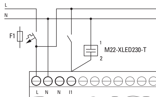
Obr. 8: Zvýšení vstupního proudu s M22-XLED230-T
