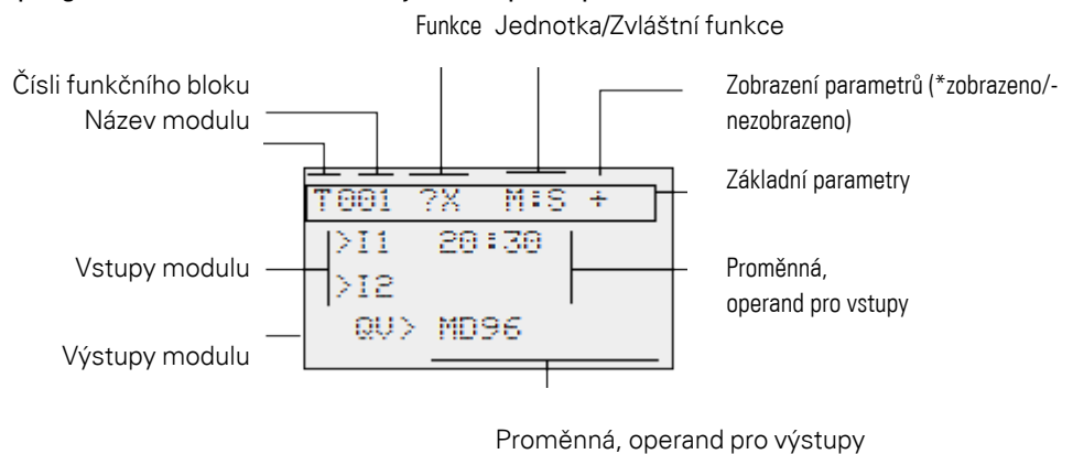
Obr. 120: Zobrazení modulů výrobce v editoru modulu
