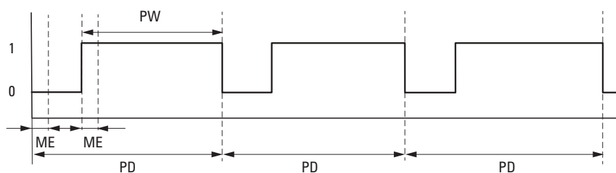
Obr. 189: Impulsy PW na vstupu modulu při SV = 3218 , ME = 93 ms, PD = 1000 ms
