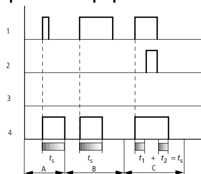
Obr. 149: Funkční diagram časového relé, podle impulsu 1
