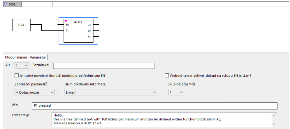
Obr. 338: Záložka modul alarmu s parametry příkladu a program FBD s modulem alarmu tlačítka P P01
