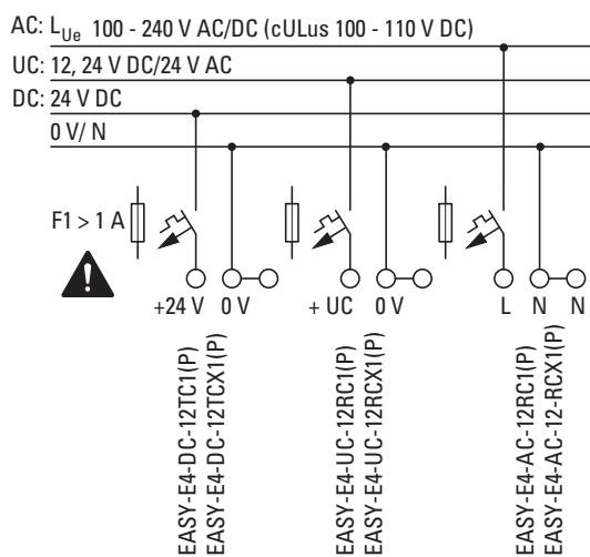
Obr. 17: Připojení napájecího zdroje základního přístroje
