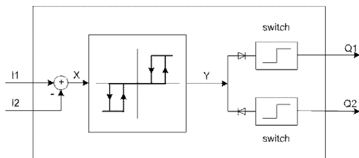
Obr. 202: Princip zapojení tříbodového regulátoru
