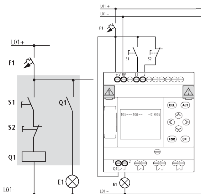
Obr. 82: Ovládání žárovek
