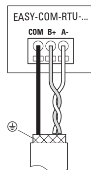
Obr. 347: EASY-COM-RTU-... Připojte výstupy
