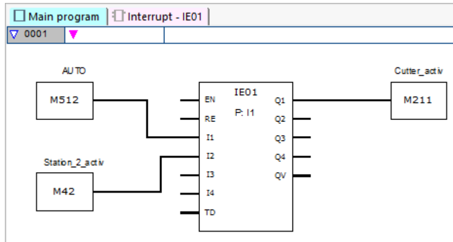
Obr. 266: easySoft 8 hlavní program řízený náběhem
