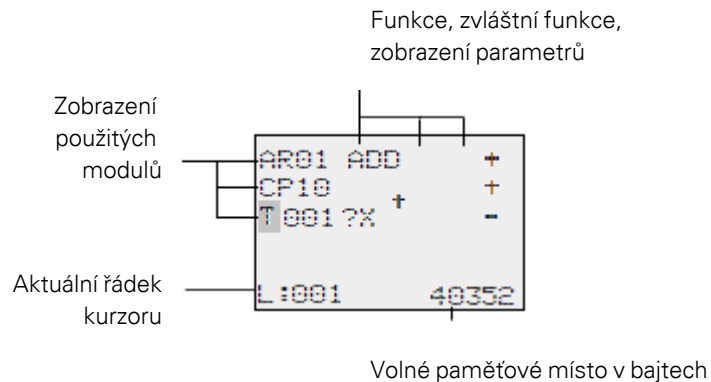
Obr. 119: Vysvětlení seznamu modulů
