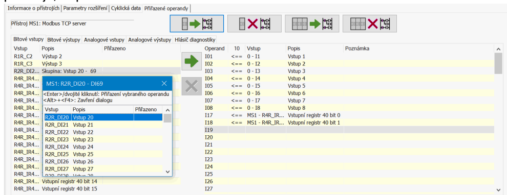
Obr. 359: Záložka Přřazené operandy bitový vstup R2R_DI20 již byl přiřazen operandu základního přístroje I19.
