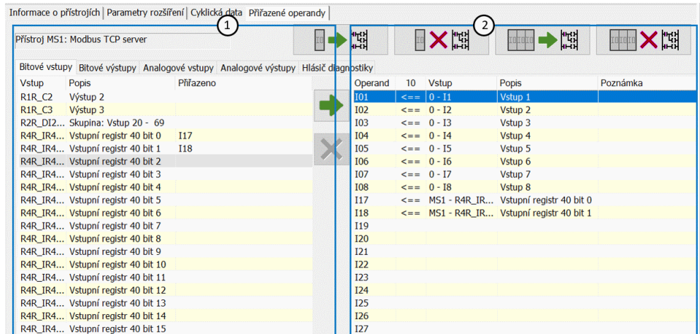
Obr. 358: Záložka Přřazené operandy podle definice FC1, FC2 a FC4; bitové vstupy R4R_IR40x0 a R4R_IR40x1 již byly přiřazeny operandům základního přístroje I17 a I18.
