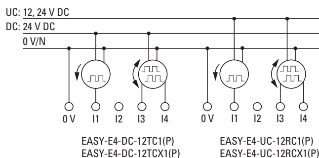
Obr. 21: připojení digitálních vstupů počítaďa
