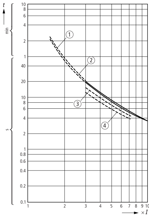
Abbildung/Figure 13: ZE-0,16/XTOMP16AC1
