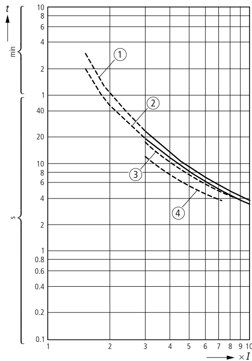
Abbildung/Figure 15: ZE-0,4/XTOMP40AC1
