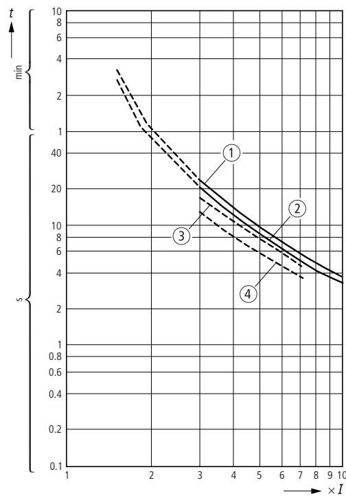
Abbildung/Figure 18: ZE-1,6/XTOM1P6AC1
