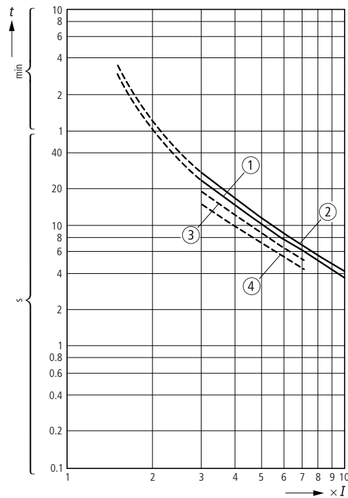
Abbildung/Figure 20: ZE-4/XTOM004AC1
