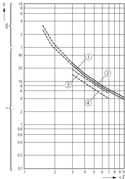
Abbildung/Figure 17: ZE-1,0/XTOM001AC1
