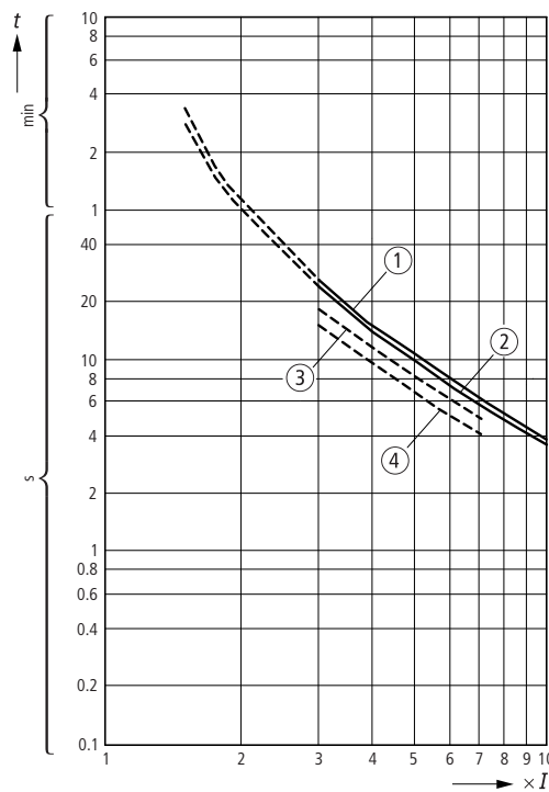
Abbildung/Figure 21: ZE-6/XTOM006AC1
