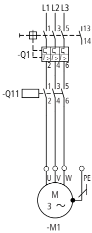
Q11 Mains contactor
