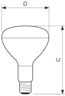
R125 IR 375W E27 230-250V CL 1CT/10
