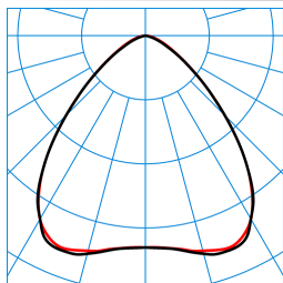
Mirona Fit 2L BS B 130-840 ETDD TX197584
