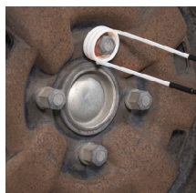
Het losdraaien van wielmoeren
