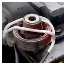
Verwijderen van een silentblock
