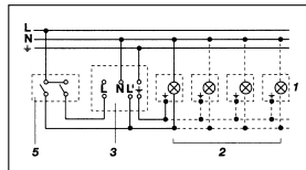
3. Liitäntä sarjakytimen välityksellä käsi- ja automaattikäyttöön
