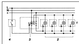
1. Valaisimet ilman nolajohdinta
