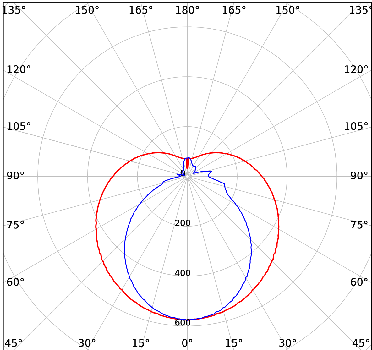
cd 3000 lm — C0-C180 — C90-C270
