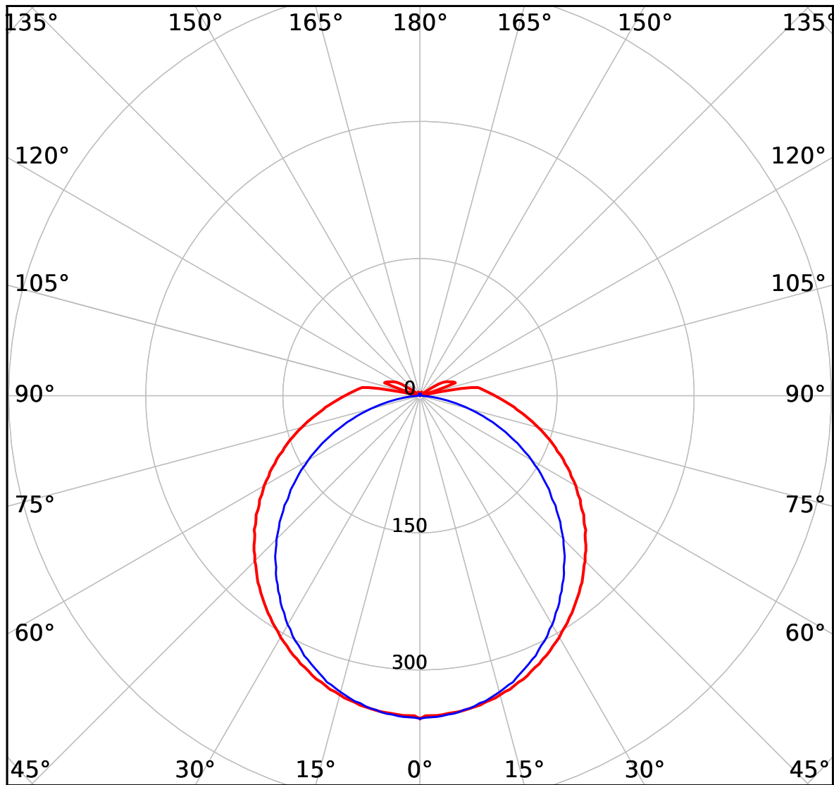
cd 1300 lm — C0-C180 — C90-C270
