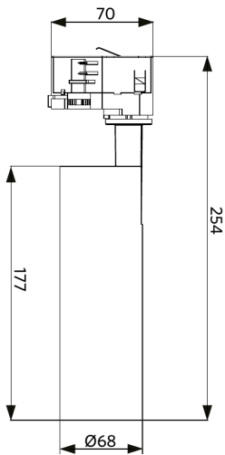
LEDSpot3C-C-CS 20W
