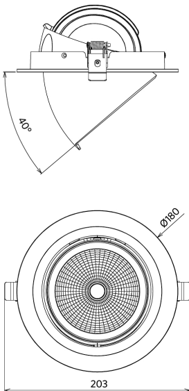
LEDspotRS-P 35W
