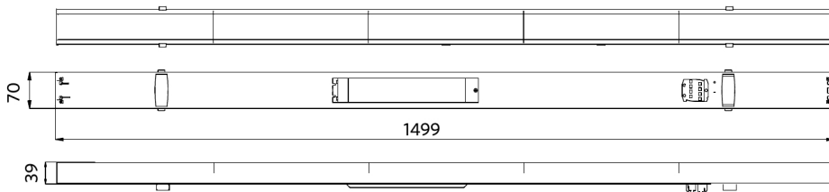
Tragschiene 8 Verbindungsstück
