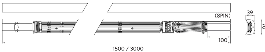
Tragschiene 8 Endstück
