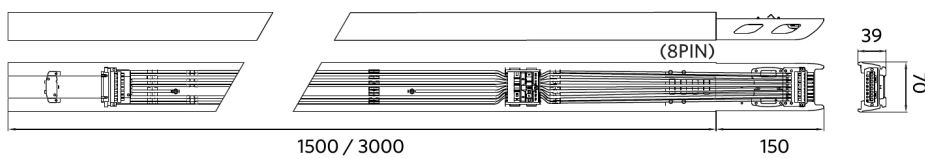
Tragschiene 8 Endstück
