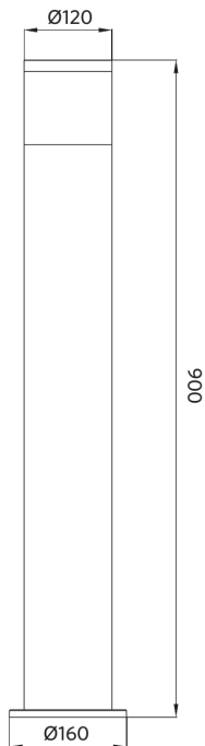
LEDBollard-P L900
