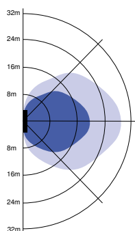
Instalação - Montado na parede Altura de instalação sugerida 1-4m
