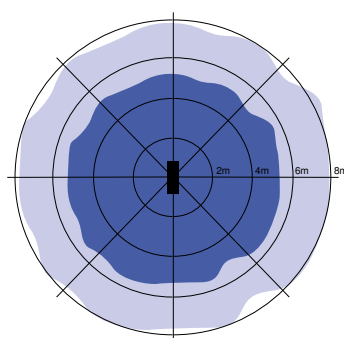
Instalação - Montado no tecto Altura de instalação sugerida 2.5-10m
