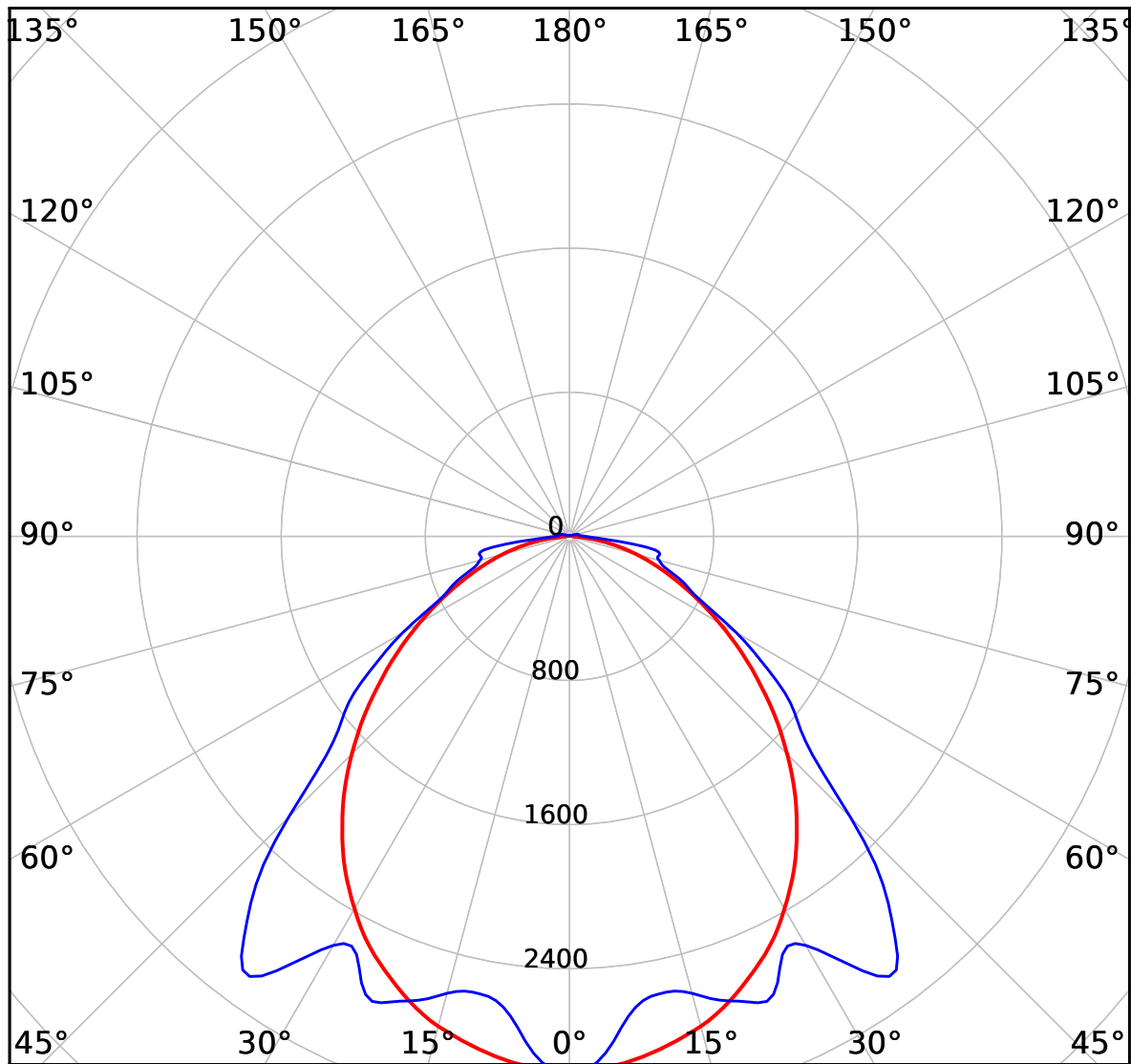
cd 8400 lm — C0-C180 — C90-C270
