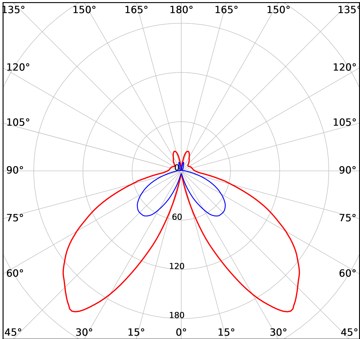
cd 620 lm — C0-C180 — C90-C270
