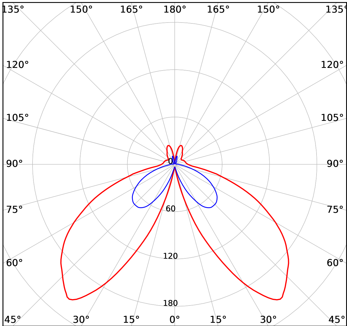
cd — C0-C180 — C90-C270 620 lm
