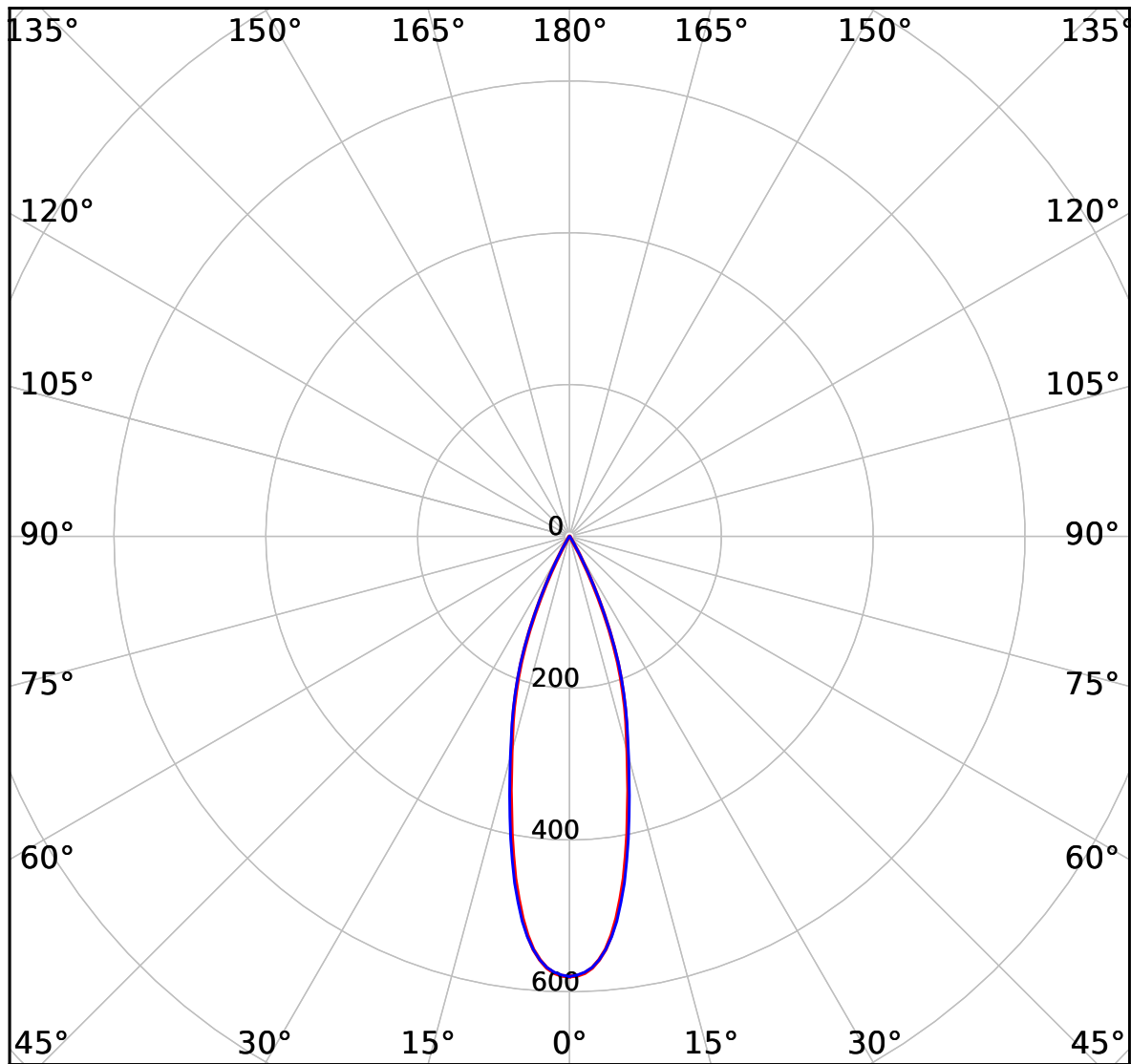
cd 180 lm — C0-C180 — C90-C270
