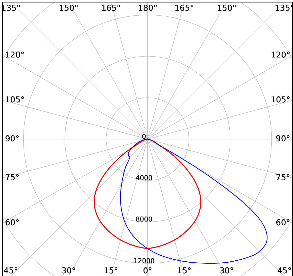
cd 28000 lm — C0-C180 — C90-C270
