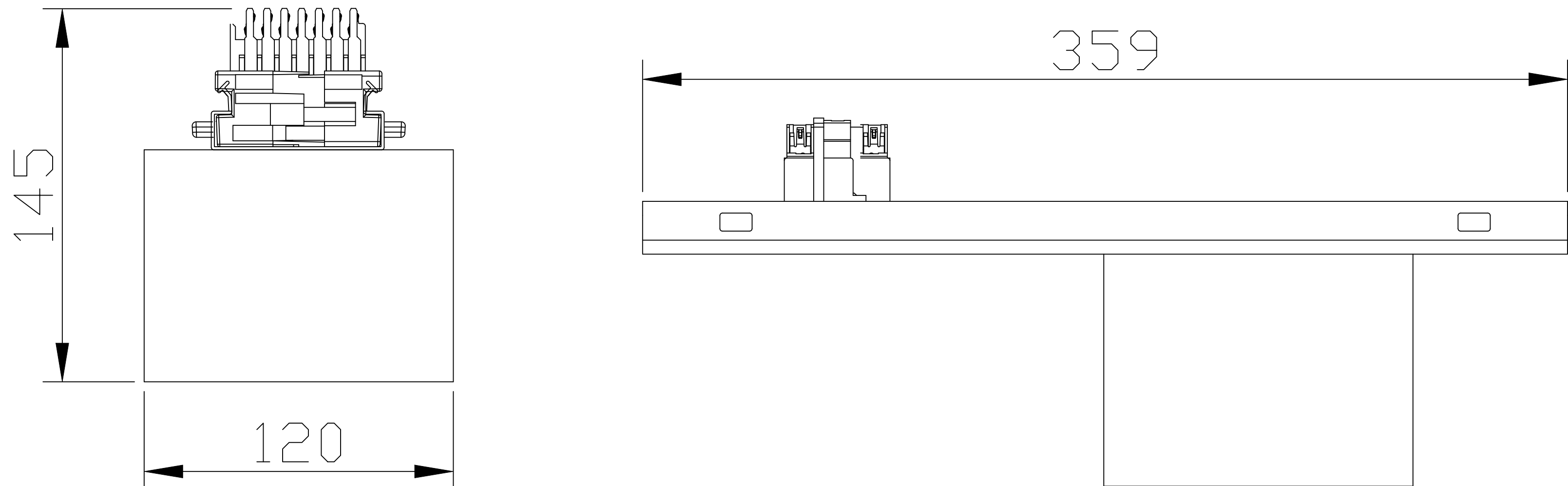
PIR Sensor Dali / DALI input
