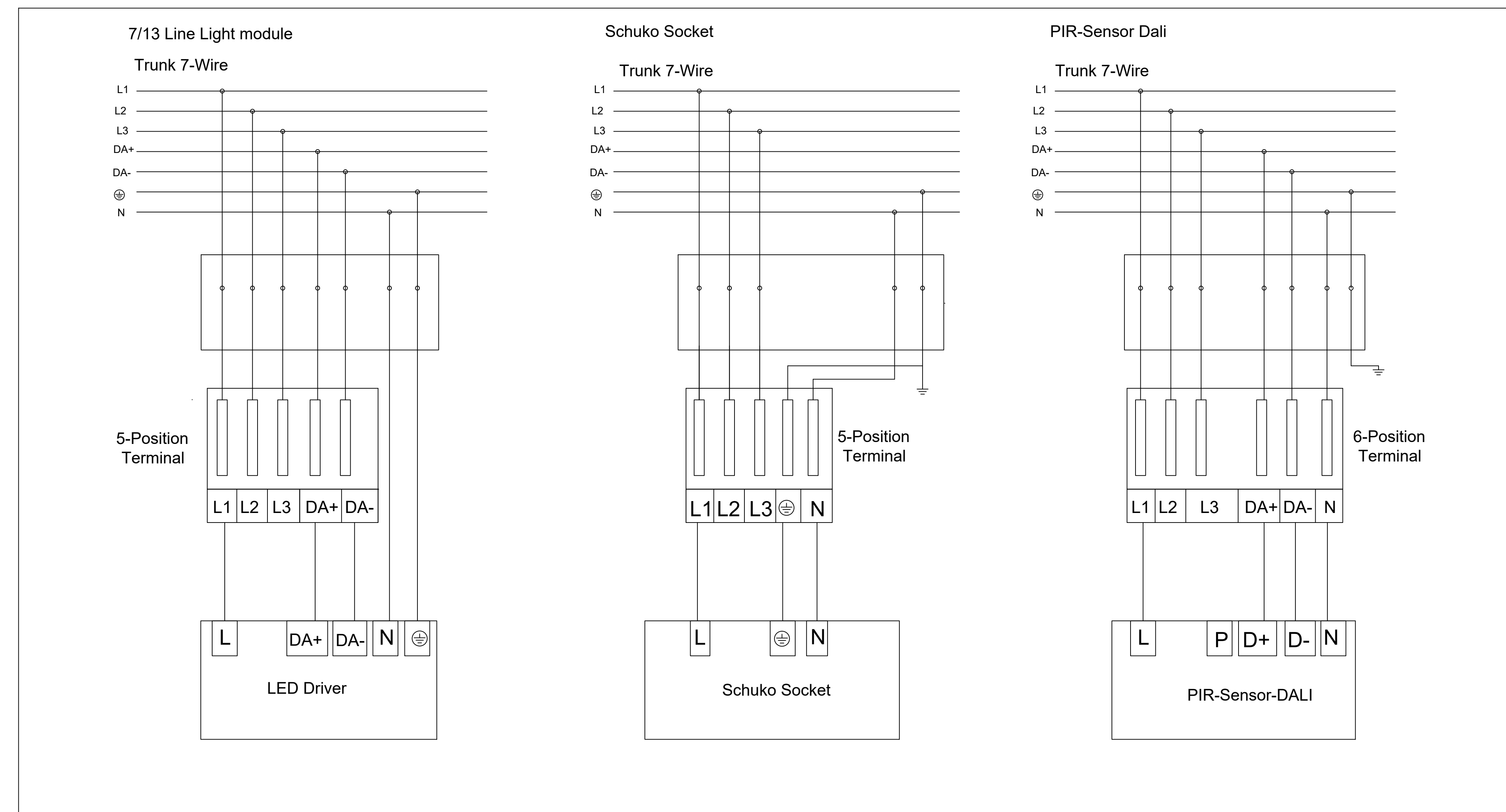
Module Wiring Schematic
