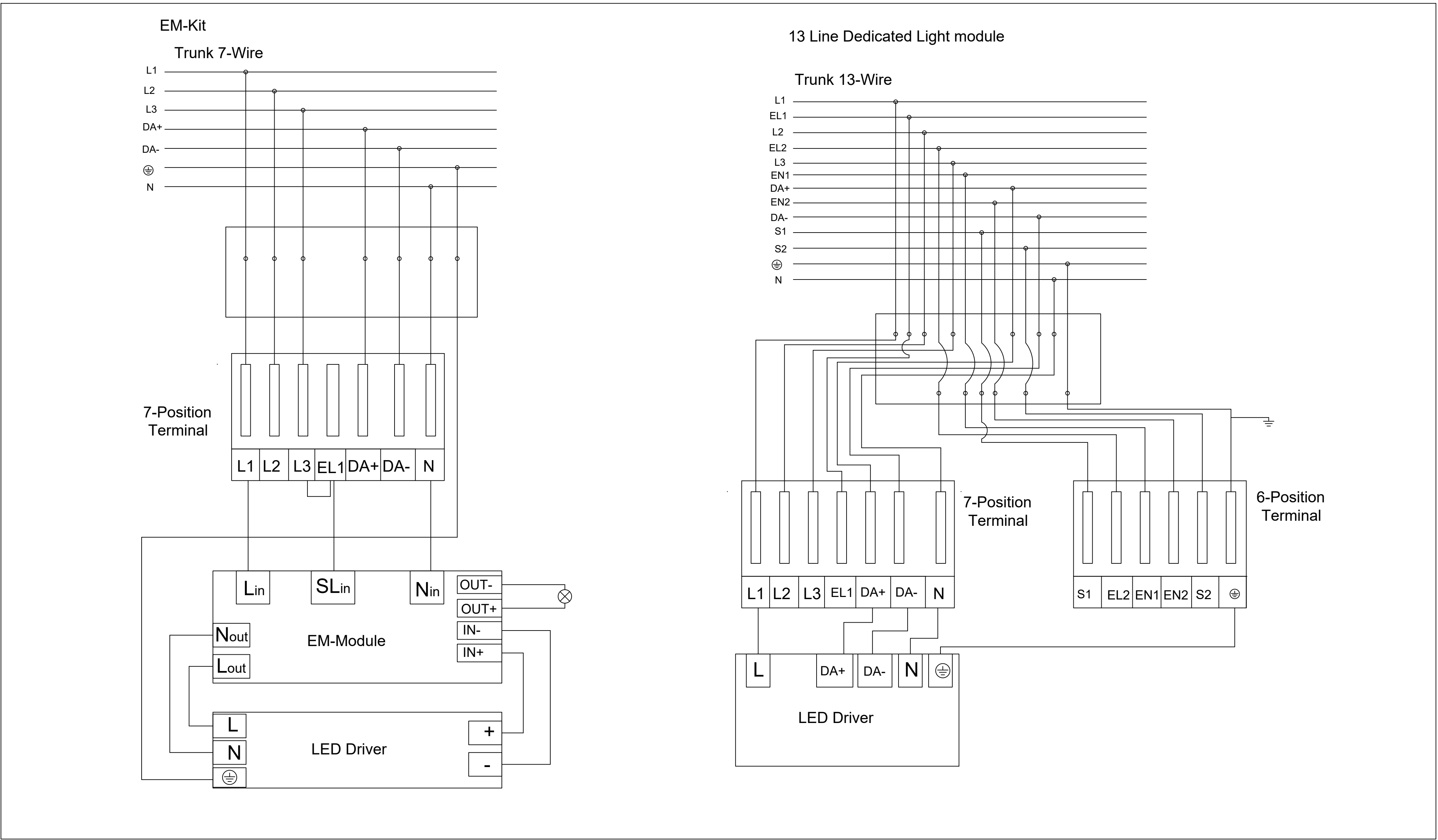
Module Wiring Schematic
