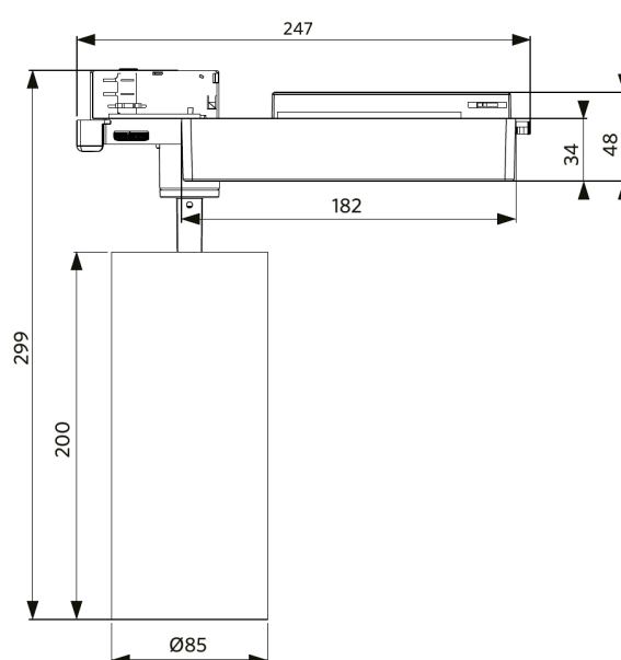
LEDspot3C-C-P 28W-BLE
