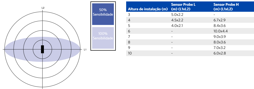
Instalação - Ceiling Mounted
