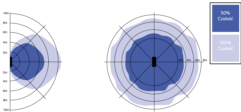
Instalacja - Montowane na ścianę Sugerowana wysokość instalacji 1.5-3m
