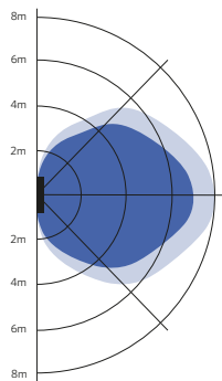
Asennus - Seinäasennus Suositeltava asennuskorkeus 1-3m
