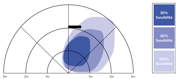
Piantana Sensore PIR e a microonde
