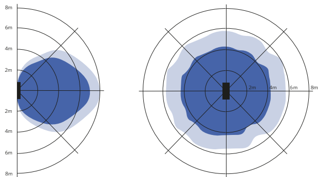
Installatie - Muur montage Aanbevolen installatie hoogte 1-3m
